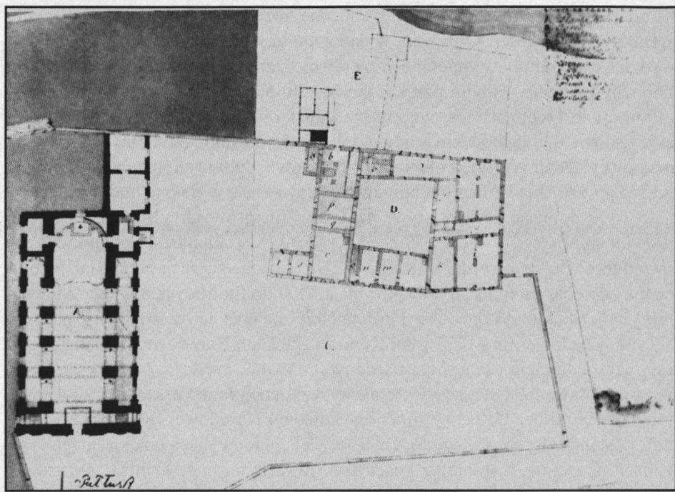
Ryc. 3. Stanisław Zawadzki, plan budowli jezuickich w Pułtusku – fragment. Rzut kościoła, kolegium i szkoły. Fot. w zbiorach ATJ
