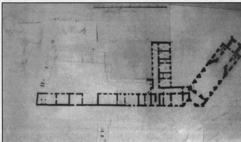
Ryc. 4. Stanisław Zawadzki, plan budowli jezuickich w Płocku – fragment. Rzut kolegium i kościoła. Fot. w zbiorach ATJ
