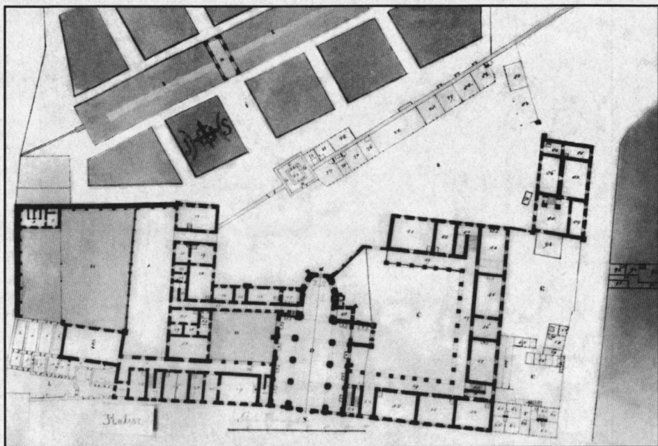
Ryc. 11. Stanisław Zawadzki, plan budowlı pojezuickich w Kaliszu – fragment. Rzut kolegium, kościoła i szkoły – parter. Fot. w zbiorach ATJ
