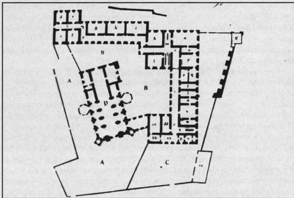
Ryc. 24. Stanisław Zawadzki, plan budowli pojezuickich w Sandomierzu – fragment. Rzut kolegium, szkoły i kościoła – parter. Fot. w zbiorach ATJ
