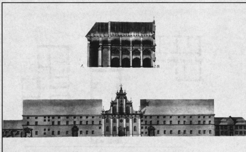
Ryc. 14. Stanisław Zawadzki, plan budowli jezuickich w Kaliszu – fragment. Elewacje kolegium, kościoła i szkoły oraz przekrój kościoła. Fot. w zbiorach ATJ
