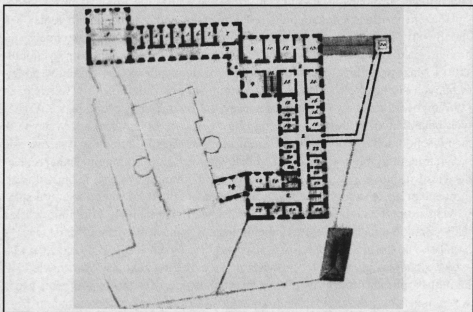
Ryc. 25. Stanisław Zawadzki, plan budowli pojezuickich w Sandomierzu – fragment. Rzut kolegium, szkoły i kościoła – pierwsze piętro. Fot. w zbiorach ATJ
