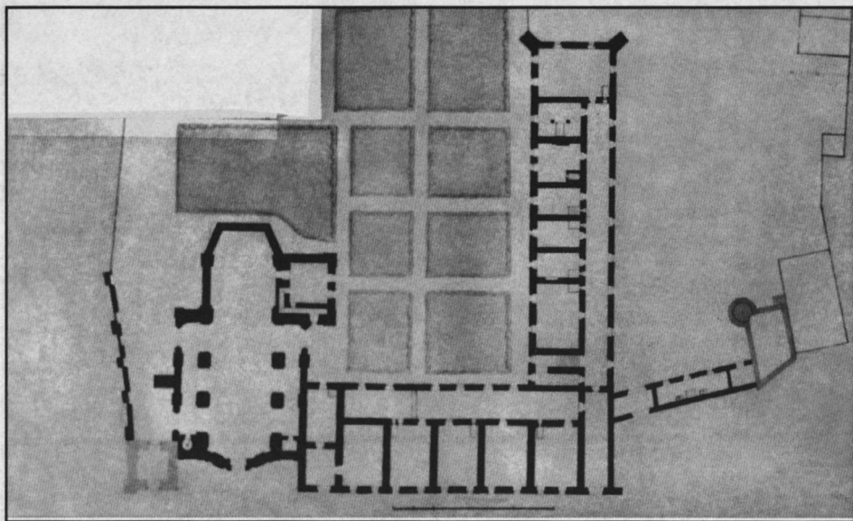
Ryc. 17. Stanisław Zawadzki, plan budowli pojezuickich w Rawie Mazowieckiej – fragment. Rzut kościoła, kolegium i szkoły. Fot. w zbiorach ATJ
