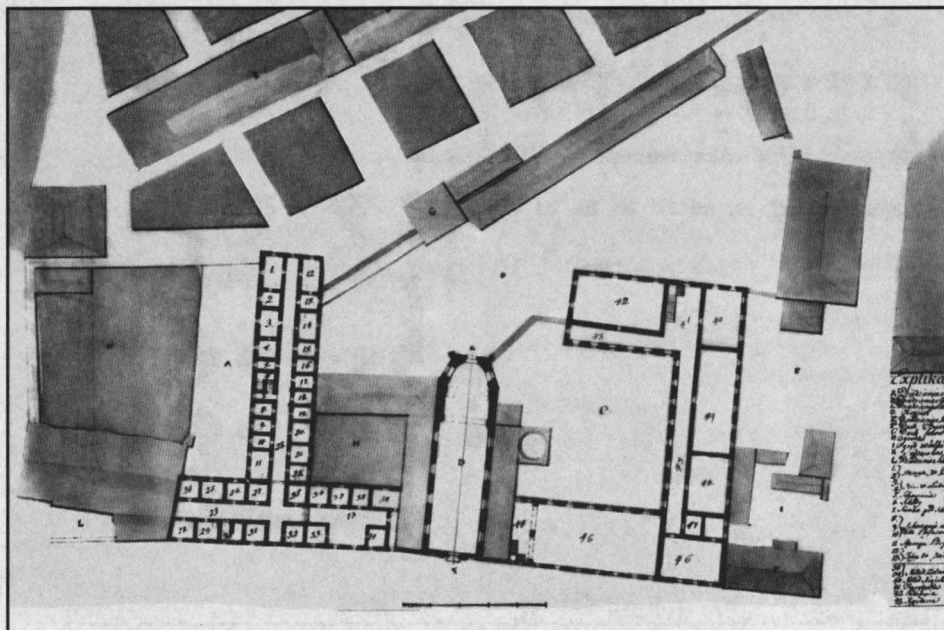
Ryc. 13. Stanisław Zawadzki, plan budowli jezuickich w Kaliszu – fragment. Rzut kolegium, kościoła i szkoły – drugie piętro. Fot. w zbiorach ATJ
