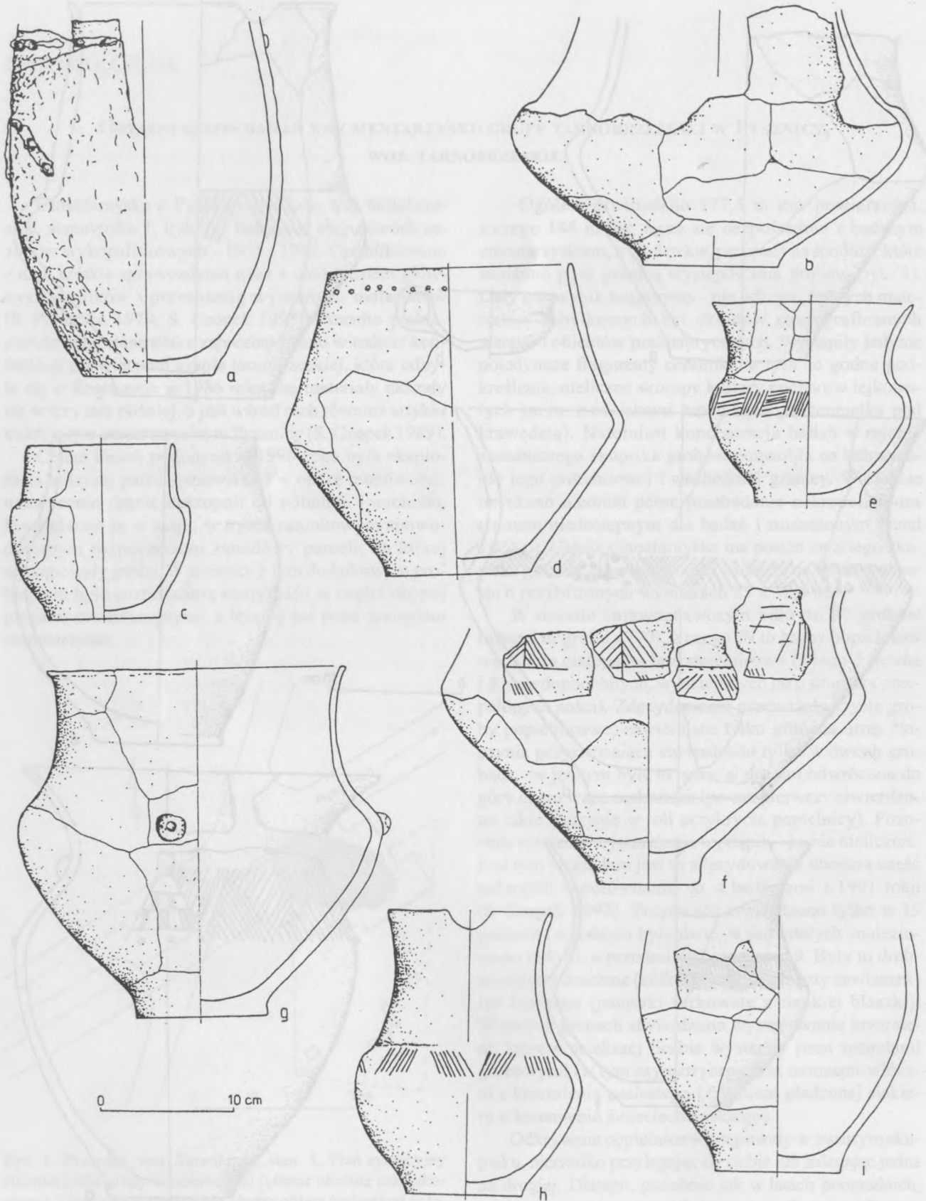
Ryc. 3. Pysznica, woj. Tarnobrzeg, stan. 1. Ceramika z grobów wyeksplorowanych w 1996 r.: 729 (a), 718 (b), 765 (c), 736 (d), 705 (e), 737 (f), 714 (g), 702 (h), 724 (i).
