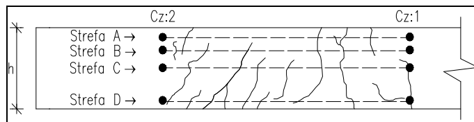
Rys. 3. Zarysowana lewa strona belki żelbetowej z zaznaczeniem stref badań, rozciągnięte włókna dolne. Cz: 1 – czujnik nr 1, Cz: 2 – czujnik nr 2
