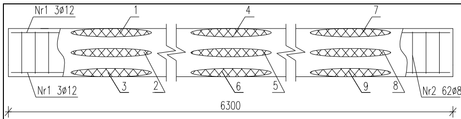
Rys. 1. Zbrojenie belki żelbetowej z zaznaczeniem stref badań przed zarysowaniem
