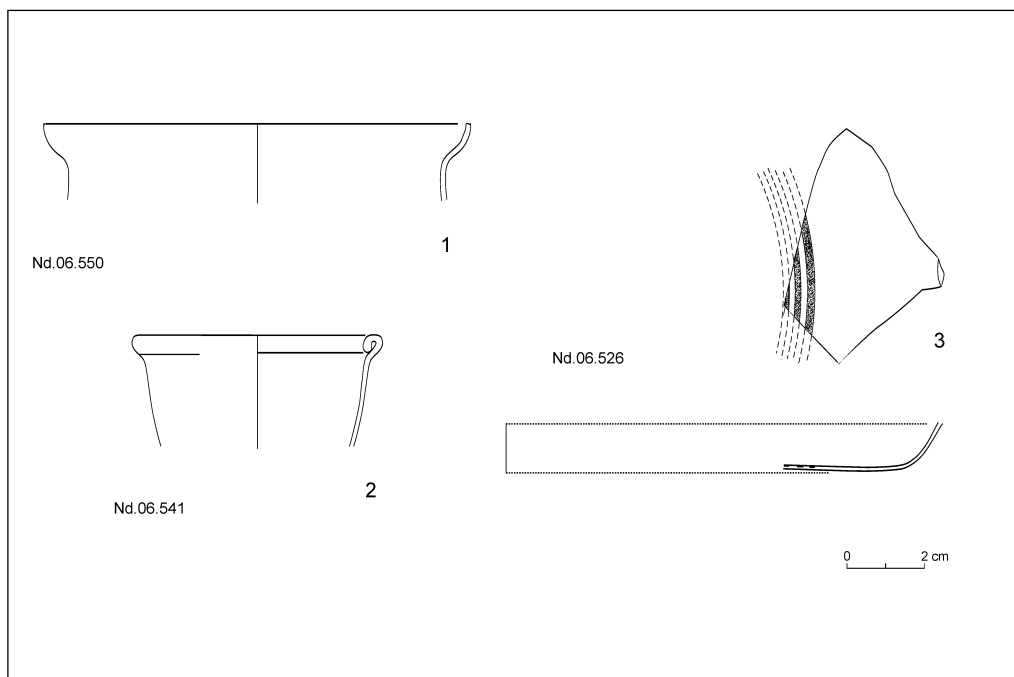
Fig. 3. Fond d'une assiette plate avec une décor gravé (1) et deux bols (2,3) (Dessin M. Mossakowska-Gaubert)
