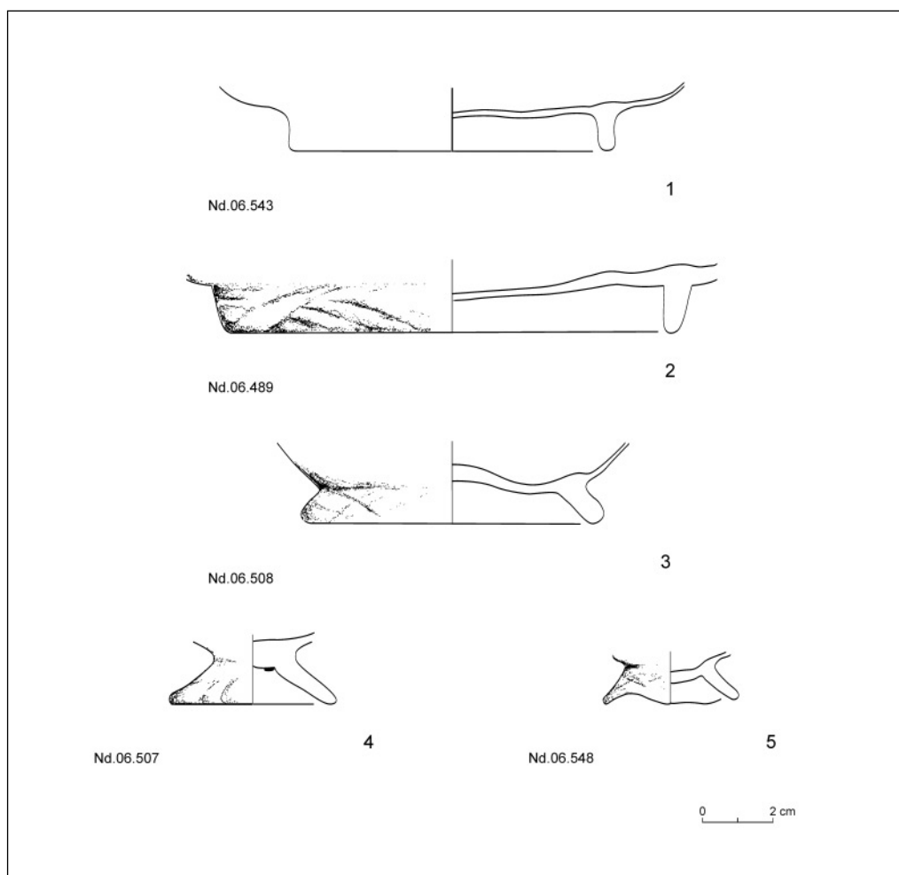
Fig. 2. Pieds d'assiettes ou de bols (Dessin M. Mossakowska-Gaubert)
