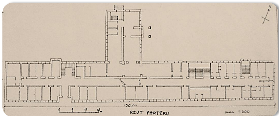
Rzut parteru budynków przy ul. Konstytucyjnej 81/83 (obecnie ul. Legionów) – stan po 1945 r. (Rejonowy Zarząd Infrastruktury Bydgoszcz Oddział w Łodzi, teczka podstaw prawnych nr 387, k. 15)
