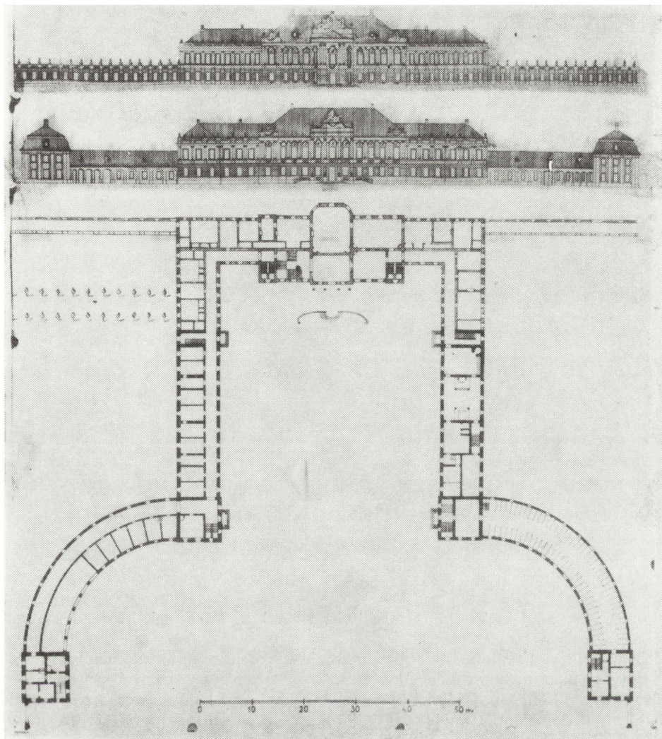
Ryc. 3. Trzy rysunki projektu pałacu w Końskich
