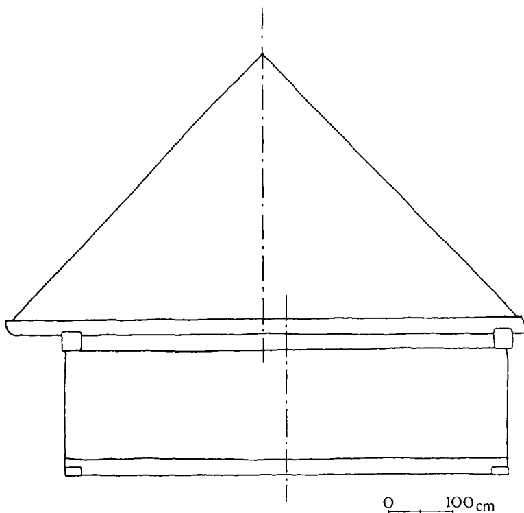
Ryc. 13. Schemat dachu asymetrycznego
