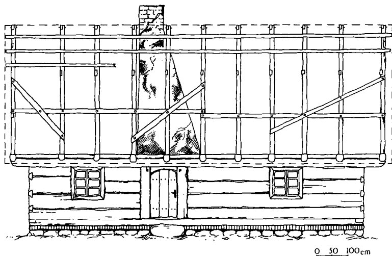
Ryc. 14. Dach krokwiowo-jętkowy chałupy ołęderskiej (1823 r.) z 60 centymetrowym nadwieszeniem w szczytach. Od frontu, szeroki okap wysunięty poza lico ściany wzdłużnej. Nowy Tomyśl (stan z 1885 r.). W 1986 r. obiekt przeniesiony do WPE
