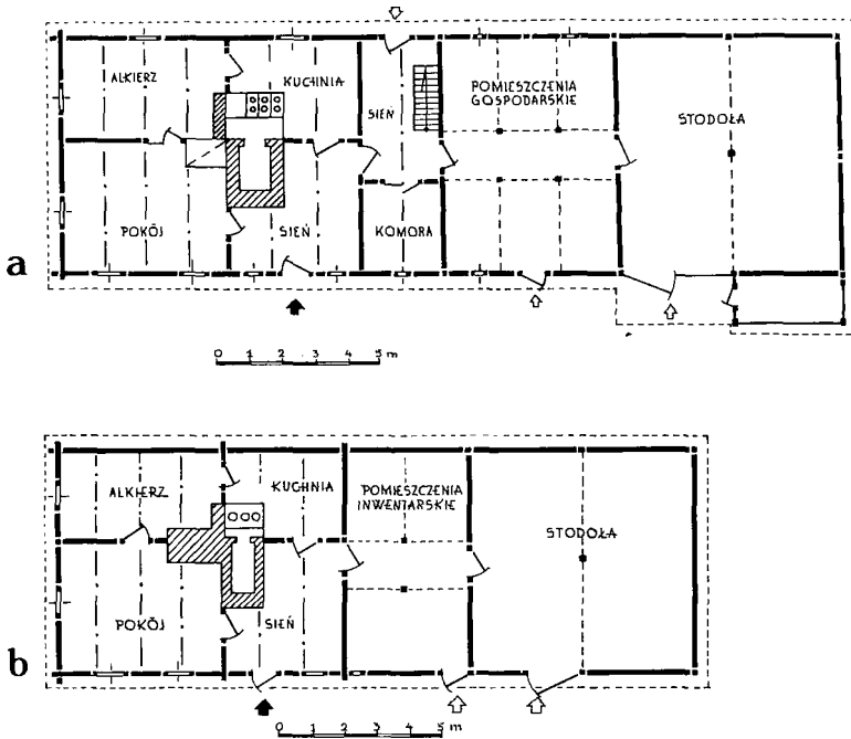
Ryc. 11. Rzuty przyziemia chałup ołędzskich nad Bugiem a) Mościce Dolne nr 14; b) Mościce Dolne nr 33, woj. białkopodlaskie (wg J. Górnika 1971, s. 33 i 34)
