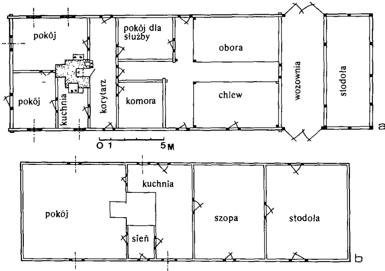
Ryc. 10. Rzuty przyziemia chałup ołęderskich w dolinie środkowej Wisły: a) Troszyn, woj. plockie; b) okolice Świecia, woj. bydgoskie (wg W. Marchlewskiego 1988, s. 508)
