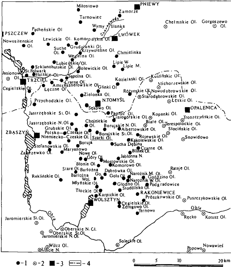
Ryc. 1. Osady ołeĀderskie powstałe na terenie niecki nowotomyskiej pod koniec XVIII wieku (por. W. Rusiński 1947, mapa). 1 — osady ołeĀderskie na terenie niecki; 2 — osady ołeĀderskie poza niecką; 3 — inne miejscowości; 4 — granice powiatów
