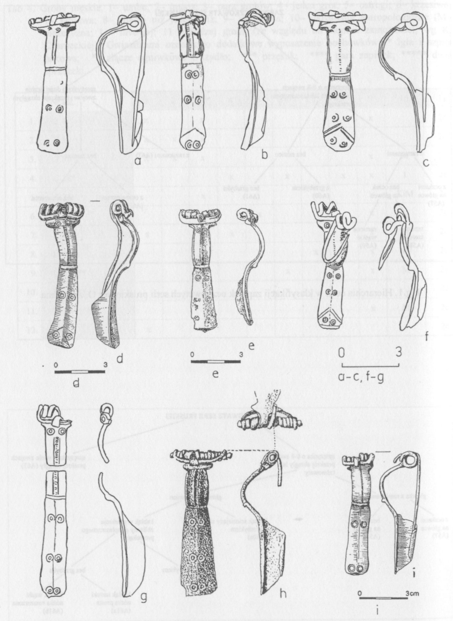
Fig. 3. Zapinki typu A57 (a-g) oraz A58/59 (h,i): a – Kat. 10.3; b – Kat. 10.5; c – Kat. 14.1; d – Kat. 17.14; e – Kat. 17.17; f – Kat. 18.3; g – Kat. 20.2; h – Kat. 2.1.a; i – Kat. 7.23.b; wg GRZYMKOWSKI 1986 (a), ZIEMIŃSKA-ODOJOWA 1999 (d,e), SZMIT 1923 (h), DĄBROWSKA 1997 (i)
