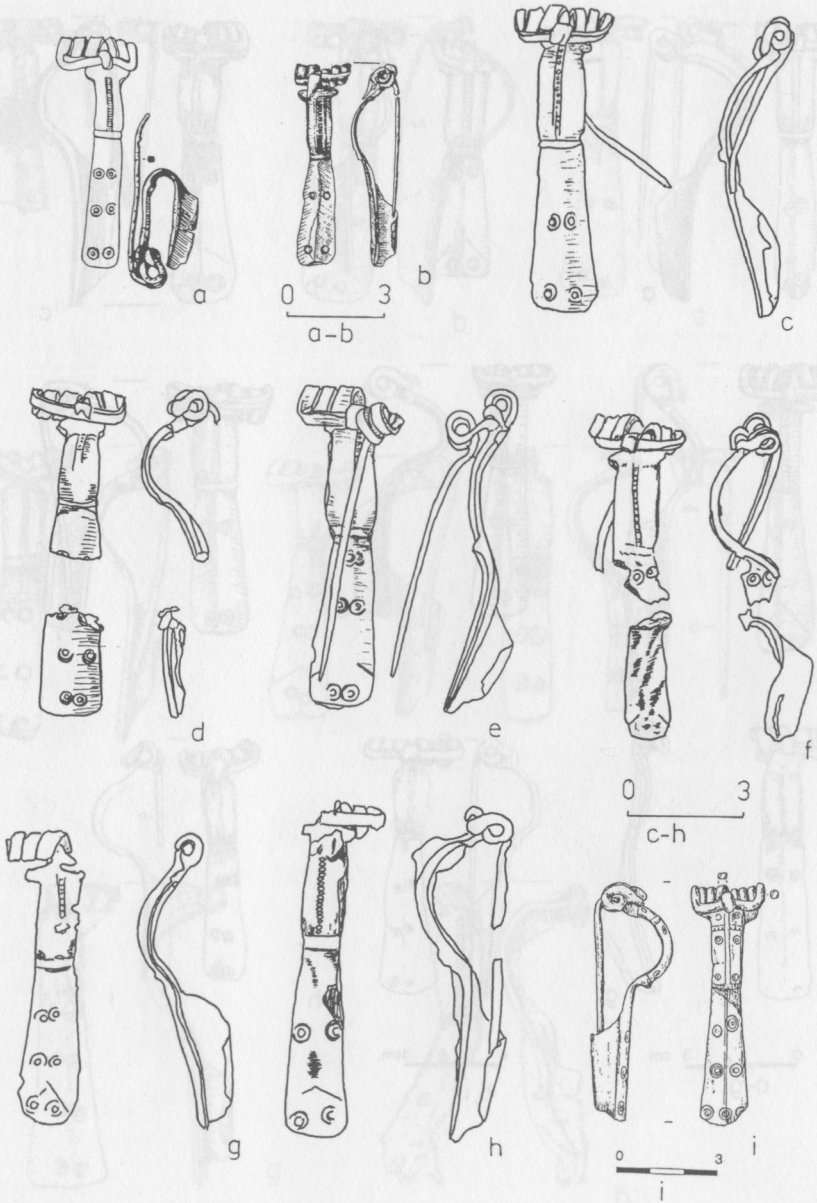
Fig. 4. Zapinki typu A58/59; a – Kat. 7.24a; b – Kat. 7.25; c – Kat. 10.4b; d – Kat. 10.12b; e – Kat. 13.3a; f – Kat. 14.1b; g – Kat. 14.5a; h – Kat. 14.6a; i – Kat. 15.6; wg: DĄBROWSKA 1997 (a, b), GRZYMKOWSKI 1986 (g), ANDRZEJOWSKI 1998 (i)
