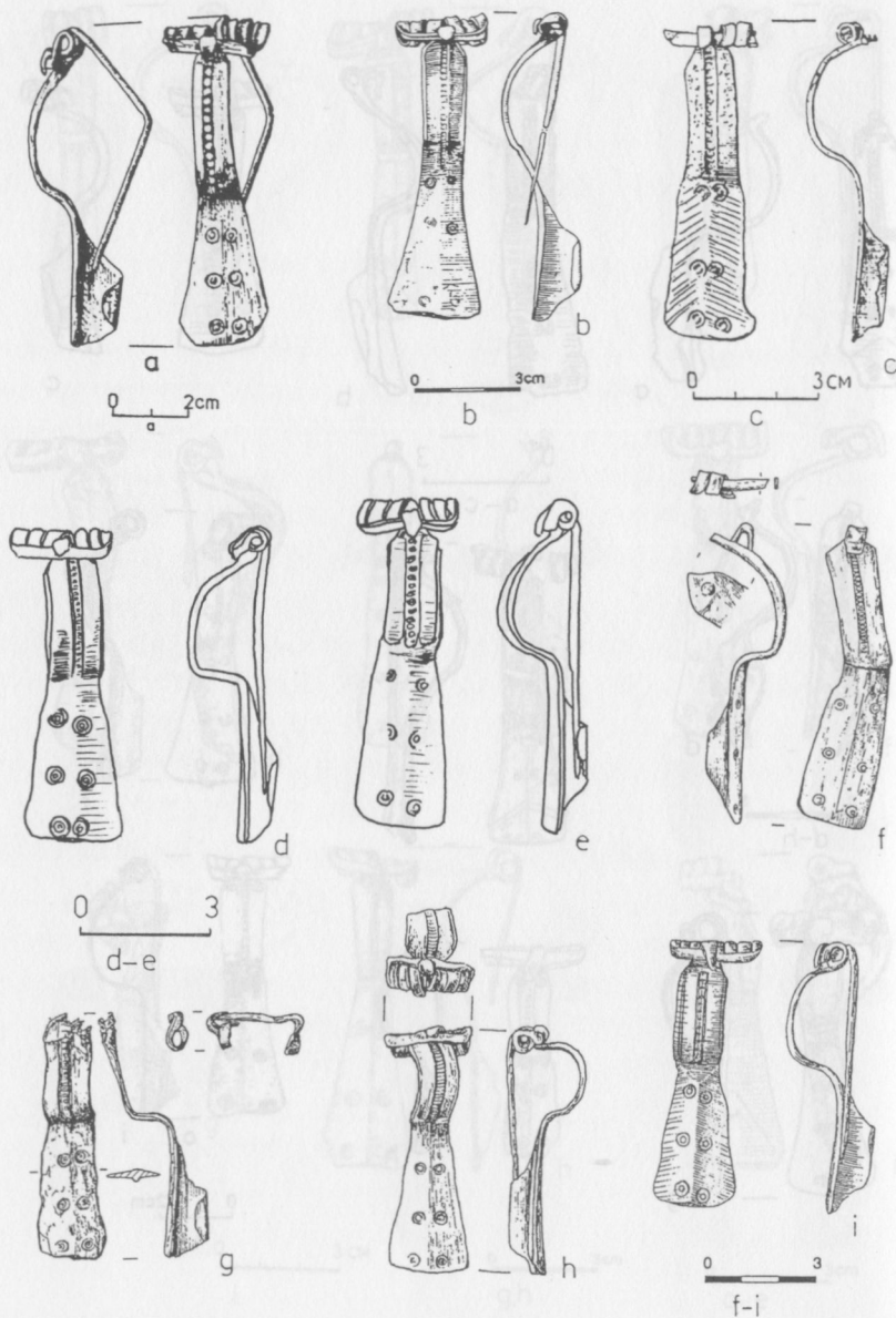
Fig. 11. Zapinki typu A61a: a – Kat. 3.4; b – Kat. 7.3; c – Kat. 8.3.a; d – Kat. 14.13; e – Kat. 14.15; f – Kat. 15.9; g – Kat. 15.18; h – Kat. 17.15.a; i – Kat. 17.20; wg: NIEWĘGŁOWSKI 1991 (a), DĄBROWSKA 1997 (b), DĄBROWSKA 1973b (c), ANDRZEJOWSKI 1998 (f,g), ZIEMIŃSKA-ODOJOWA 1999 (h,i)
