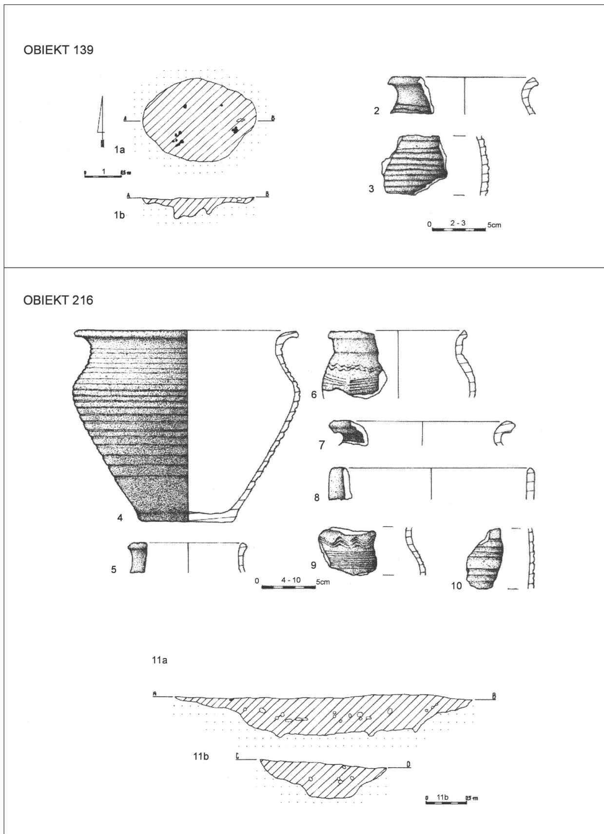
Fig. 3. Rusiec st. II gm. Nadarzyn. 1a, b – plan i profil obiektu nr 139; 2-3 – ceramika z wypełniska ob. 139; 4-10 – ceramika z wypełniska ob. 216; 11a, b – plan i profil obiektu nr 216
