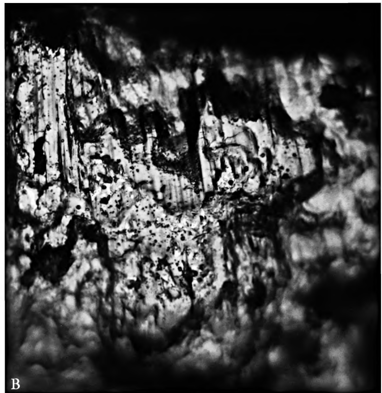
Ryc. 2. Materiały eksperymentalne: 1 – narzędzie do obróbki krzemienia; 2 – narzędzie do obróbki hematytu. A, B – ślady mikroskopowe, pow. \times 200 (ob. \times 10 ) (rys. P. Rozbiegalski, fot. K. Pyzewicz).
