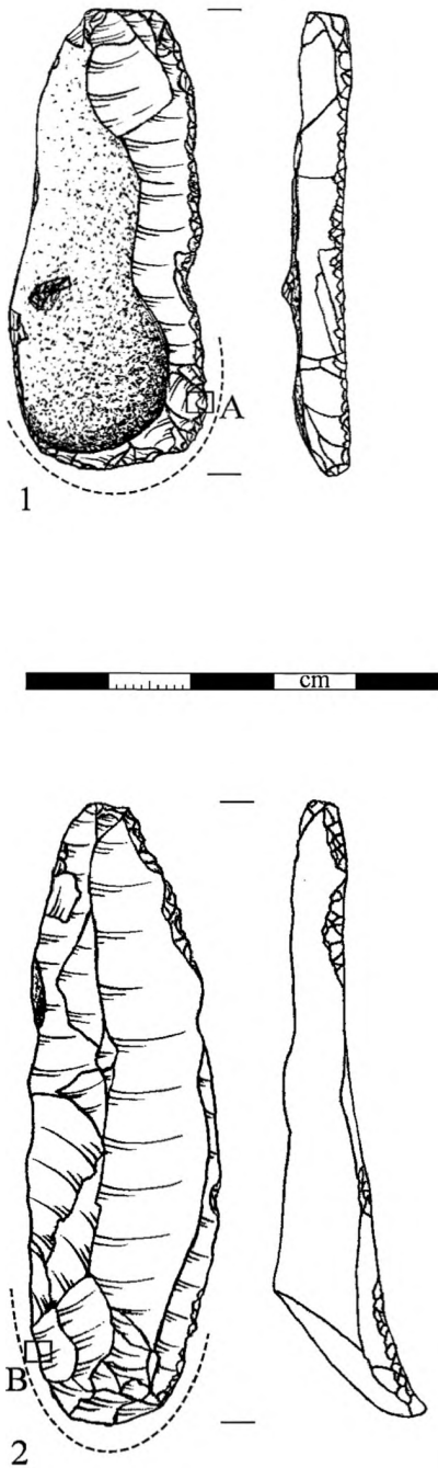
Ryc. 3. Materiały eksperymentalne: 1 – narzędzie do obróbki wapienia; 2 – narzędzie do obróbki piaskowca. A, B – ślady mikroskopowe, pow. \times 200 (ob. \times 10 ) (rys. P. Rozbiegalski, fot. K. Pyżewicz).
