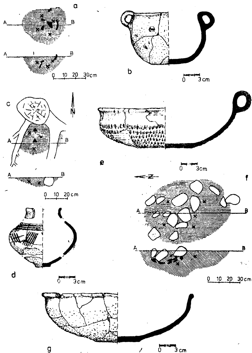
Grób nr 7: a — plan płaski i przekrój, b — baniaste naczynie z dwoma uchami; grób nr 8: c — plan płaski i przekrój, d — fragmenty niewielkiego naczynia o esowatym profilu, zdobionego grupami linii rytych, e — misa z uchem, zdobiona dołkami paznokciowymi; grób nr 9: f — plan płaski i przekrój, g — misa
