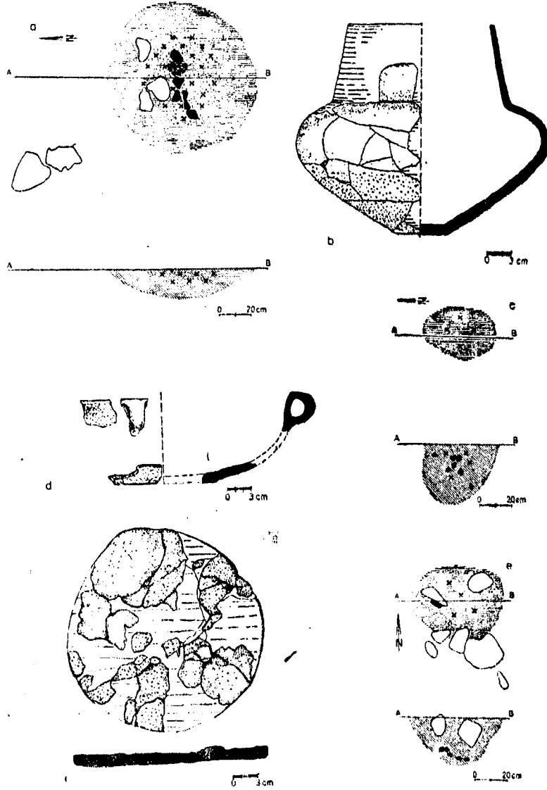
Grób nr 15: a — plan płaski i przekrój, b — naczynie dwustożkowate o zaokrąglonym załamie i stożkowato zwężającej się szyjce; grób nr 16: c — plan płaski i przekrój, d — fragmenty miski z uchem; grób nr 17: e — plan płaski i przekrój, f — fragmenty płaskiego talerza
