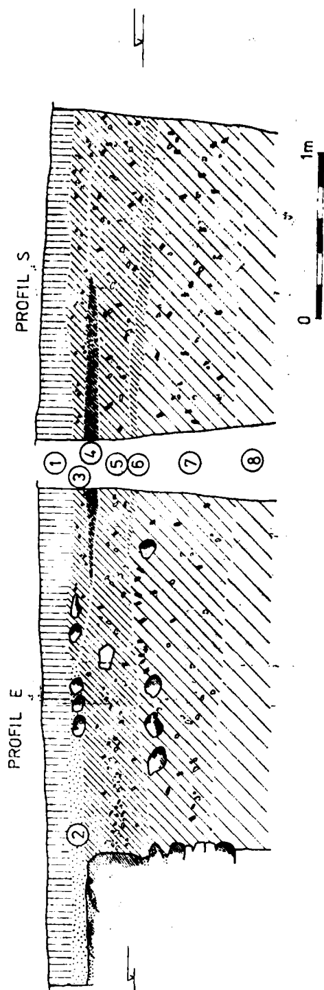
Rys. 7. Profile wschodni i południowy wykopu II. 1 — współczesny humus, 2 — piasek nasypowy, 3 poziom gliny z rumoszem, 4 — glina z węglami, 5 — brunatna glina z cegłą i nielicznymi węglami, 6 — poziom przepalanej gliny — klepiska (?), 7 — jasnobrunatna glina z węglami i drobnymi ceglami, 8 — całec, żółta, zwalowa glina
