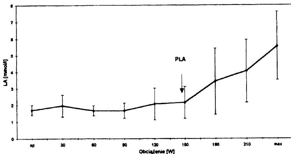
Ryc.1 Zmiany stężenia mleczanu (LA) we krwi podczas wysiłku o stopniowo wzrastającej intensywności w zależności od obciążenia ( \bar{x} \pm SD ) ↓ - próg LA
