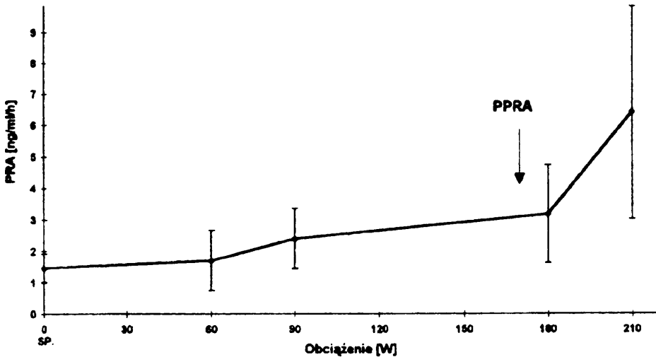
Ryc.2 Zmiany aktywności reninowej osocza (PRA) podczas wysiłku o stopniowo wzrastającej intensywności w zależności od obciążenia (x SD). ↓ -próg PRA
