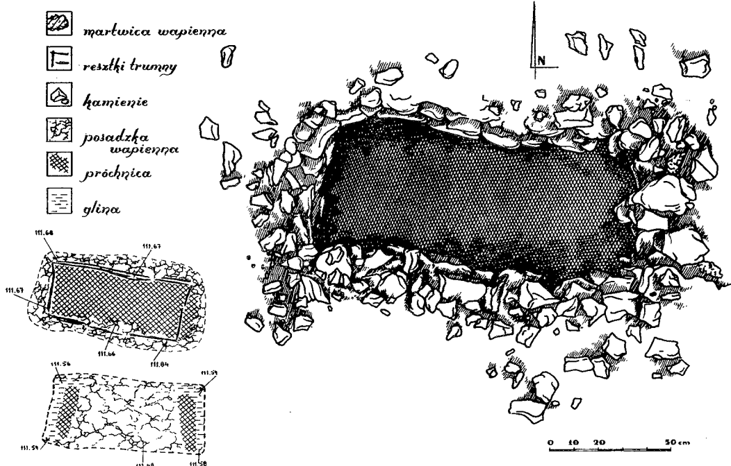
Ryc. 3. A. Grobowiec duży: rzut poziomy oraz widok na ścianę N i E grobowca. E. Grobowiec mniejszy: rzut poziomy stropu grobowca oraz jego spągu z wapienną posadzką i resztkami trumny
