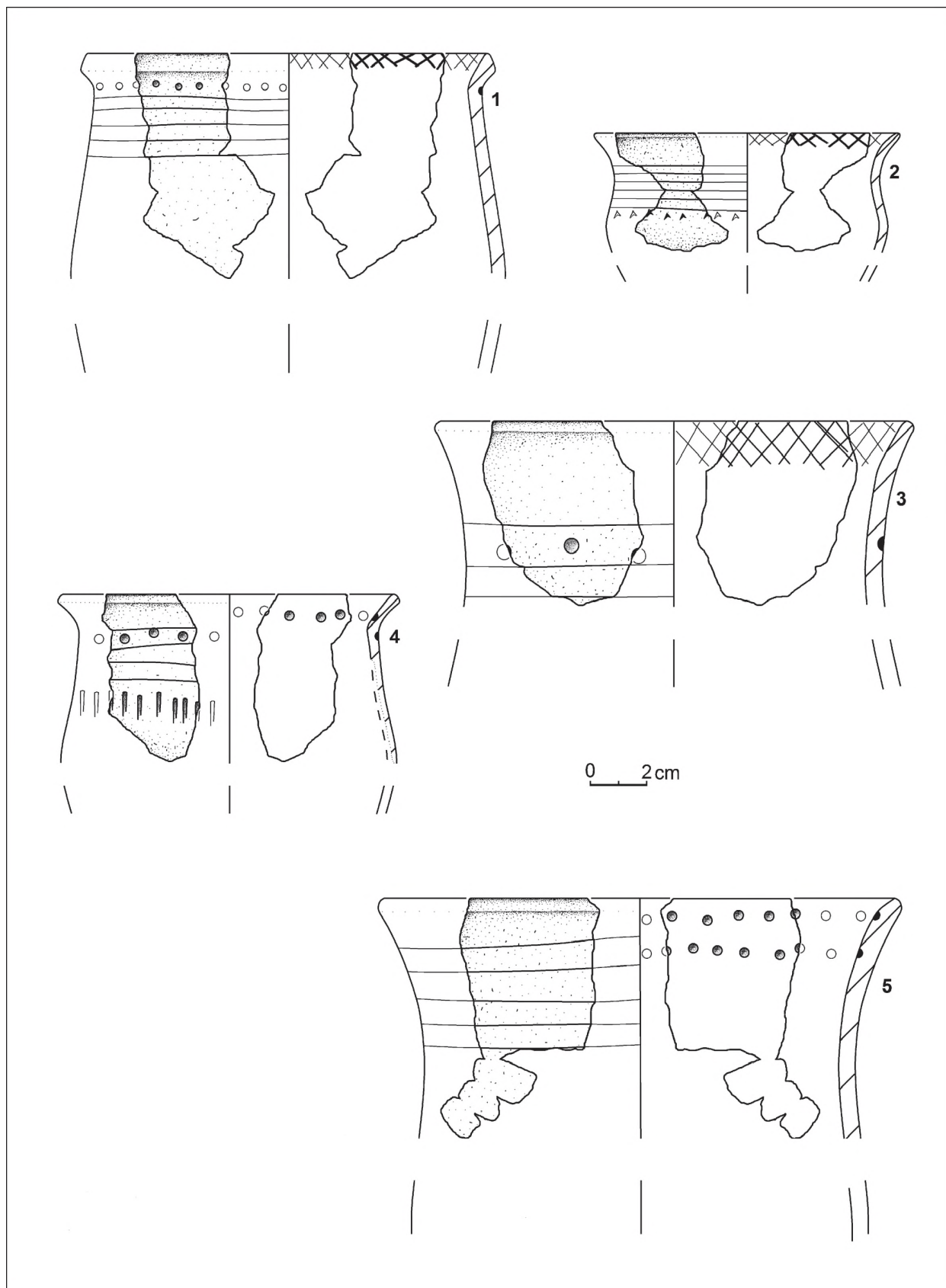
Ryc. 9. Suchacz, st. 1, gm. Tolkmicko. Wybór ceramiki o cechach iwieńsko-trzcinnieckich z warstwy kulturowej (1, 3, 4) i z jam: nr 12 (2), nr 112 (5) (rys. D. Manasterski).
