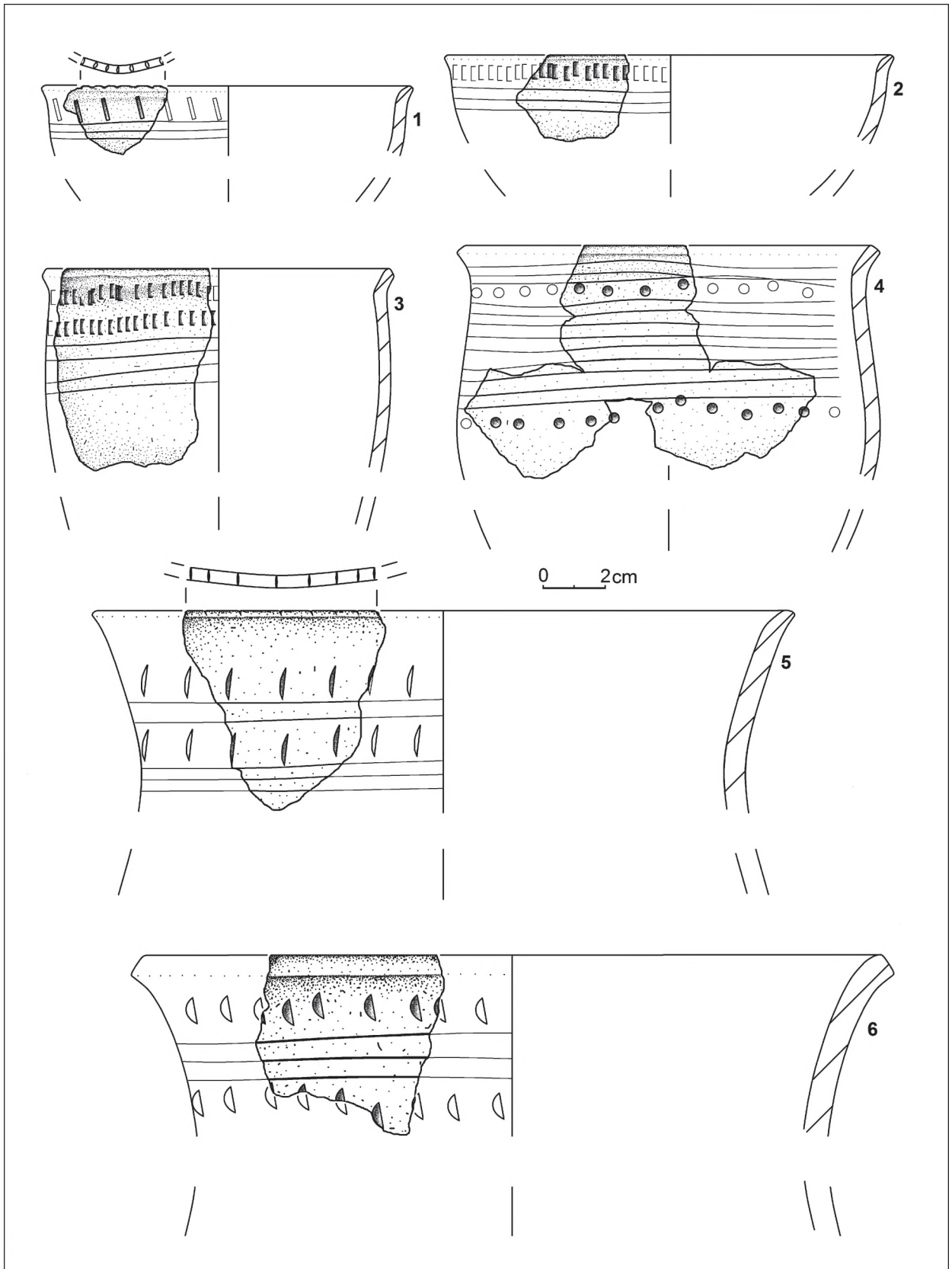
Ryc. 8. Suchacz, st. 1, gm. Tolkmicko. Wybór ceramiki o cechach iwieńsko-trzcienieckich z warstwy kulturowej (2, 5, 6) i z jam: nr 36 (2), nr 112 (3) oraz z domostwa nr III (4) (rys. D. Manasterski).
