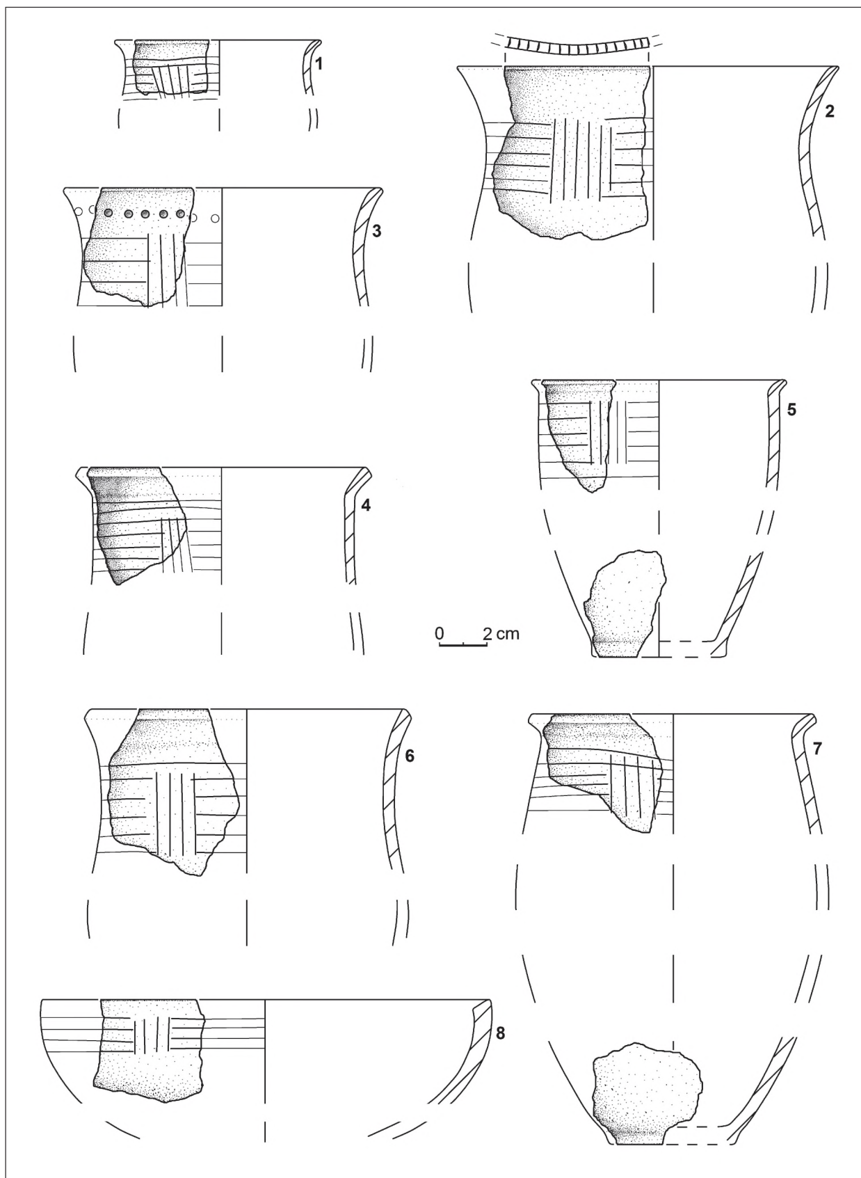
Ryc. 4. Suchacz, st. 1, gm. Tolkmicko. Wybór ceramiki o cechach iwieńsko-trzcienieckich z warstwy kulturowej (1-7) i z jamy nr 116 (8) (rys. D. Manasterski).
