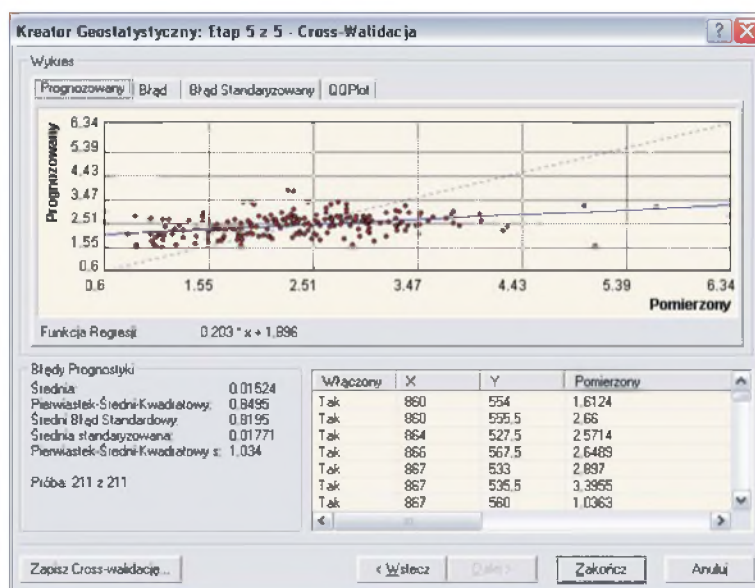
Rys. 6. Prezentacja parametrów jakościowych modelu uzyskanego przez interpolację metodą krigingu zwykłego z parametrami zoptymalizowanymi na podstawie analizy trendu
