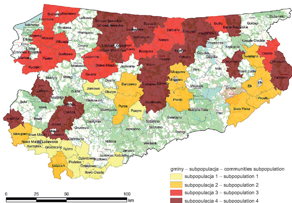
Rys. 4. Wydzielone subpopulacje metodą Warda
