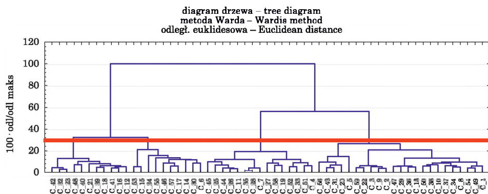
Rys. 3. Aglomeracja metodą Warda
