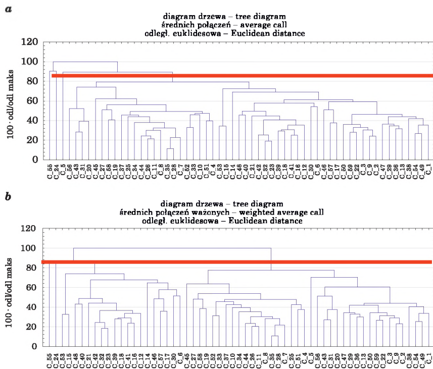
Rys. 2. Aglomeracja metodą średnich połączeń (a) i średnich połączeń ważonych (b)
