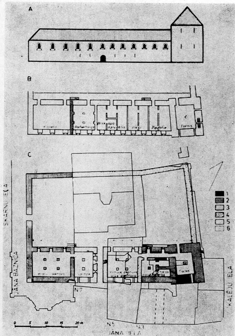
12. Zamek biskupi w Rydze. Wyniki badań architektonicznych (wg R. Zandberga, Rīgas viduslaiku nozuduso arhitekturas pieminekļu meklējumi , [w:] Muzeji un kultūras pieminekļi , Rīga 1973, s. 11, il. 11)
