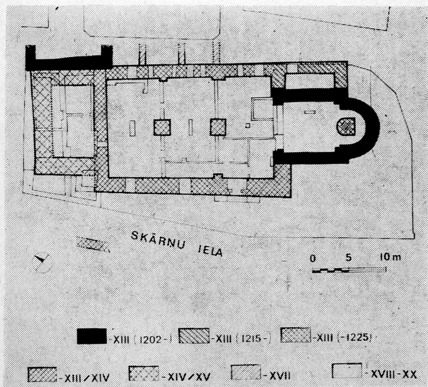
11. Kościół Świętego Ducha (św. Jerzego) wzniesiony na obszarze dawnej posiadłości kawalerów mieczowych w śródmieściu Rygi. Rozwarstwienie faz budowlanych na poziomie piwnic. Opracowanie autora na podstawie dokumentacji: B. Muzolf, Wyniki badań archeologicznych byłego kościoła św. Jerzego w Rydze ul. Skarniu 10—19, Pracownia Konserwacji Zabytków, Ryga—Łódź 1984. J. Cedro, L. Gałczewski, Wyniki badań architektonicznych dawnego kościoła zamkowego pw. Św. Jerzego w Rydze, Pracownia Konserwacji Zabytków, Ryga—Kielce 1984
