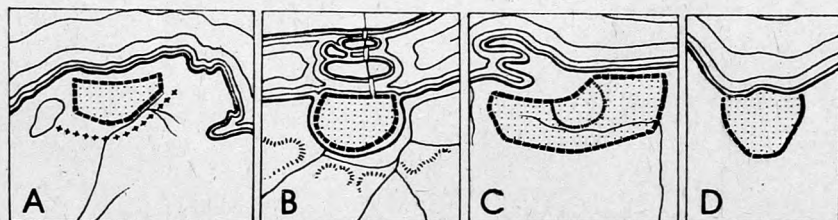
21. Przykłady wczesnośredniowiecznych portów nadbałtyckich (przerys. wg W. Filipowiak, Port wczesnośredniowiecznego Wolina , Materiały Zachodnio-Pomorskie. Muzeum Pomorza Zachodniego, t. 2, Szczecin 1956, s. 197 i n. il. 10—11, 13—14)
