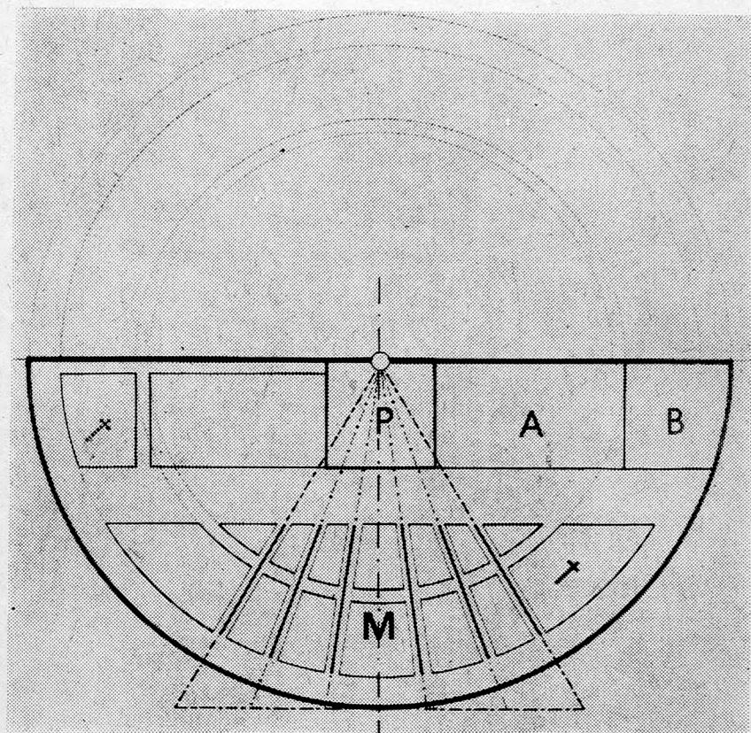
19. Rekonstrukcja tzw. „planu idealnego”, który posłużył około 1201 roku do uformowania układu przestrzennego miasta Rygi. Kompozycja geometryczna z zastosowaniem okręgu, trójkąta równoramiennego i kwadratu. Opracowanie autora
