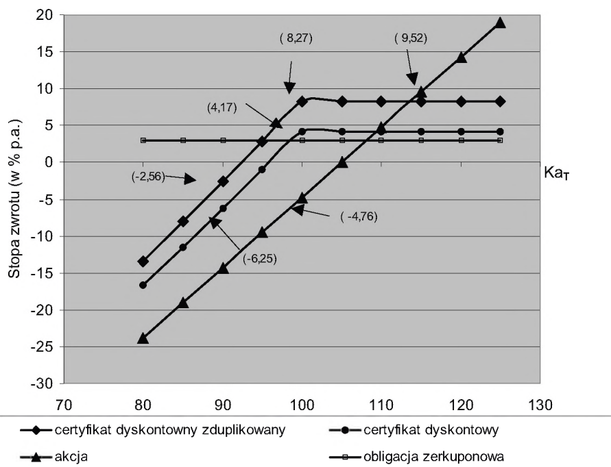
Rys.1. Profil zysków i strat z inwestycji w obligację zerokuponową, certyfikat dyskontowy, certyfikat dyskontowy zduplikowany i akcję.
