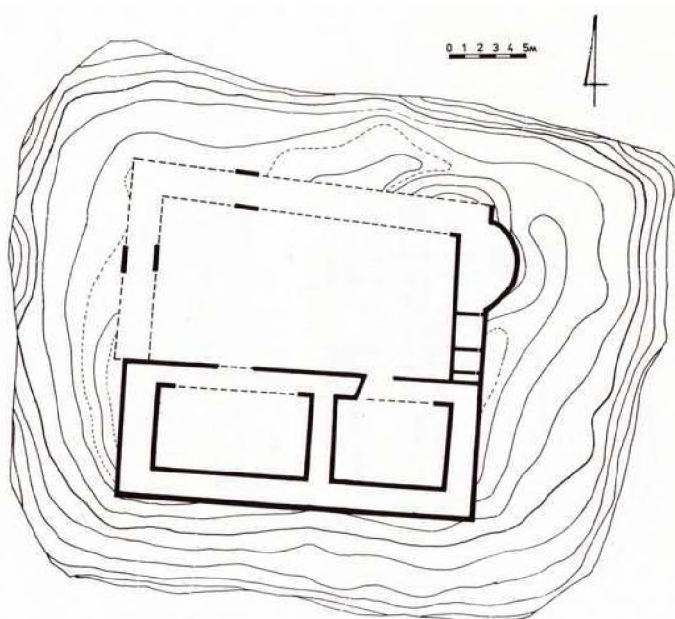
Ryc. 4. Rzut odsłoniętych fragmentów zameczku (gruba linia) w Wojsławicach
