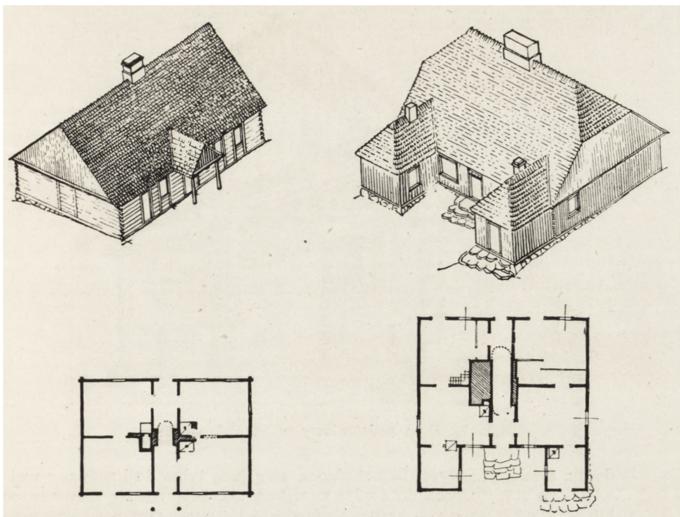
Ryc. 77 i 78. Dom z sienią na przestrzał przy ul. Nadrzecznej nr 4 w Mińsku Maz. (plan i widok na lewo); dom z alkierzami w Mińsku Maz. (plan i widok — na prawo) (Opr. autora).
