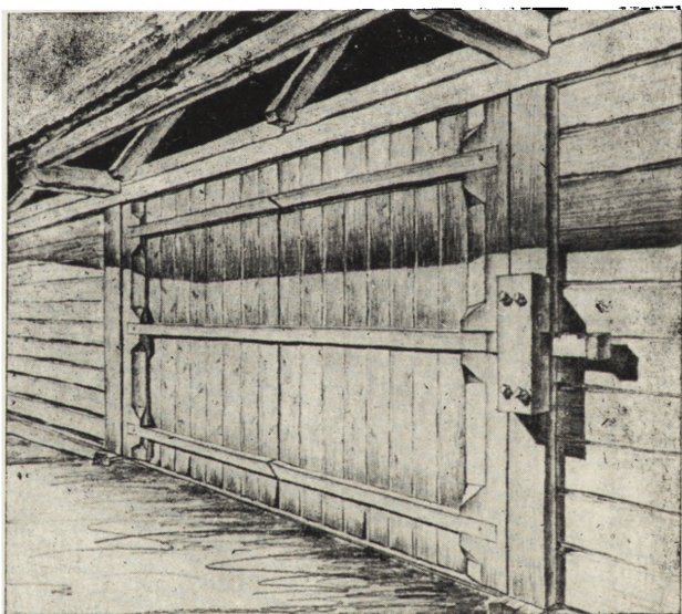
Ryc. 69. Zamek — kłoda u wierzei stodoły w Wólce Czarnińskiej (rys. autora).
