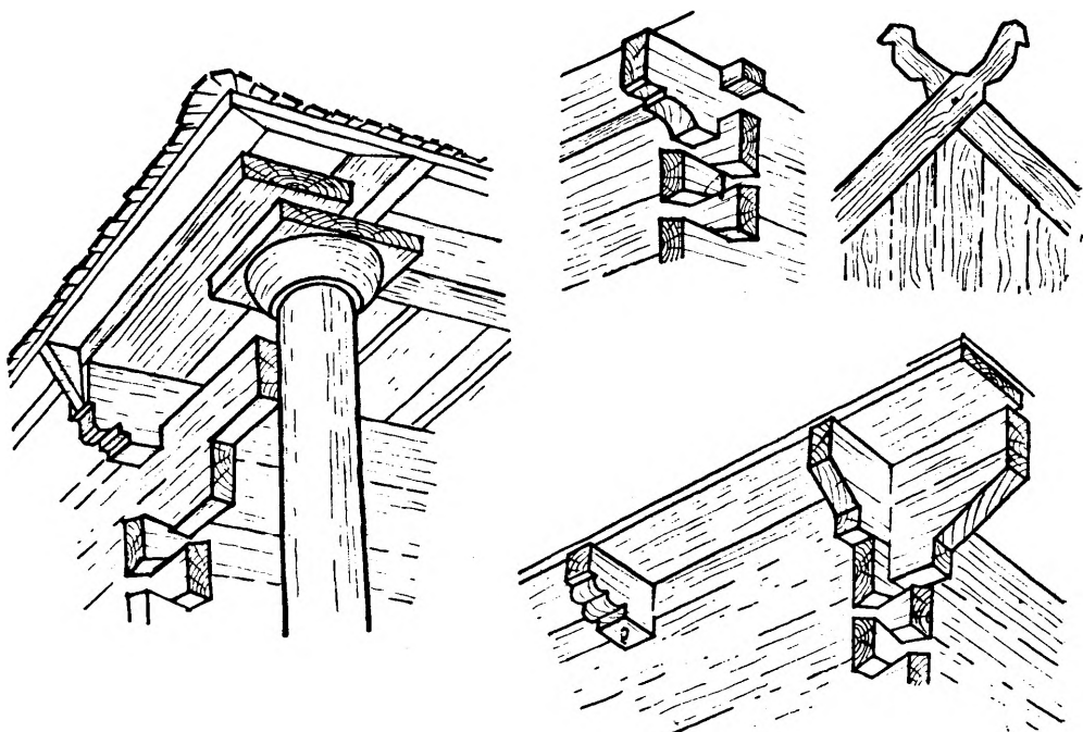
Ryc. 72—75. Szczegół narożnika domu podcieniowego w Stanisławowie (na lewo); fragment węgła domu w Latowiczu i sparogi chaty w Choszczówce Dębskiej (na prawo na górze); rysie i belka stropowa chaty w Choszczówce Dębskiej (na prawo na dole). (Opr. autora).
