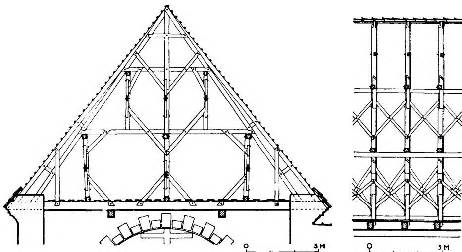
Ryc. 81 i 82. Wieżba dachowa nad prezbiterium fary w Cegłowie. Przekroje: poprzeczny (na lewo) i podłużny — fragment (na prawo). (Opr. autora).
