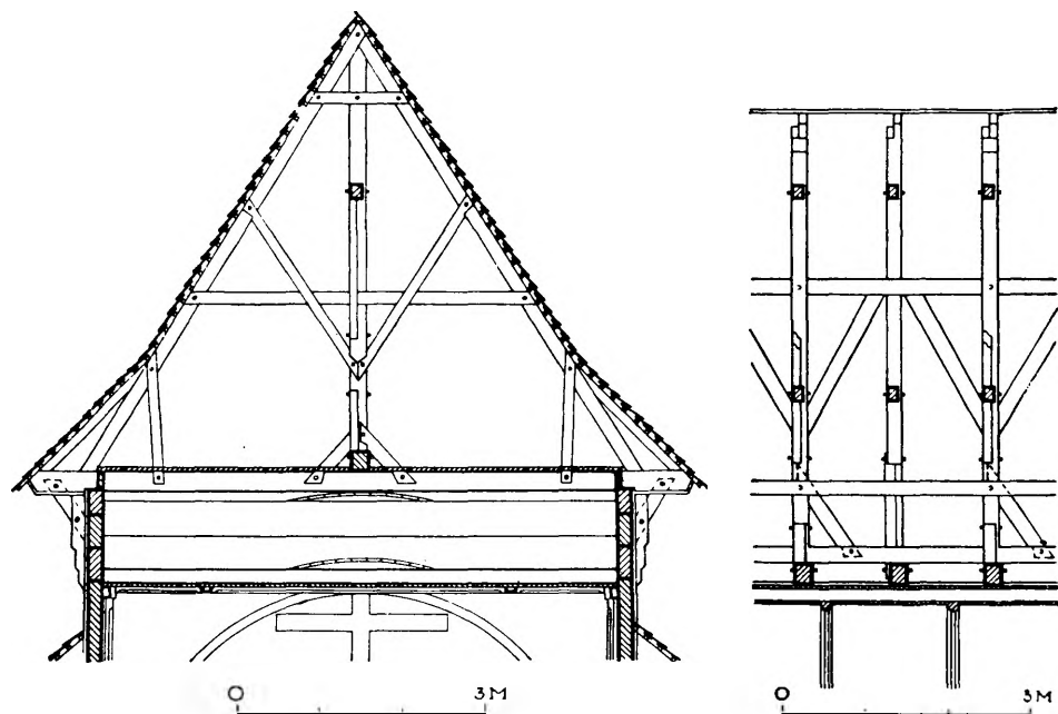
Ryc. 83 i 84. Więźba dachowa fary w Długiej Kościelnej. Przekroje: poprzeczny (na lewo) i podłużny — fragment (na prawo). Opr. autora).
