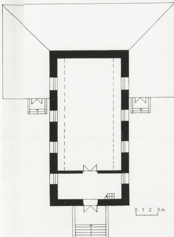
5. Dzygówka. Plan przyziemia kościoła dawniej parafialnego. Pomiar i oprac. P. Szlezzynger, 1997 r.
