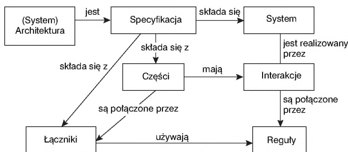
Rys. 1. Definicja Architektury Systemu według OMG MDA™. Źródło: opracowanie na podstawie C.E. Dickerson i D.N. Mavris 2010. Architecture and Principles of Systems Engineering , Boca Raton: CRC Press Taylor & Francis Group, An Auerbach Book.
