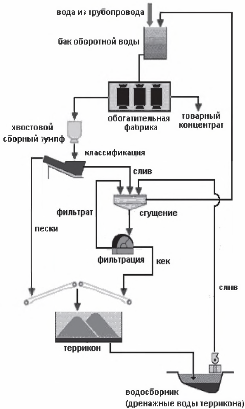
Rys. 1. Schemat ideowy technologii zwałowania odpadów w hałdach stożkowych
