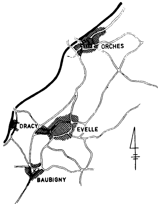
Ryc. 1. Komuna Baubigny w Burgundii
