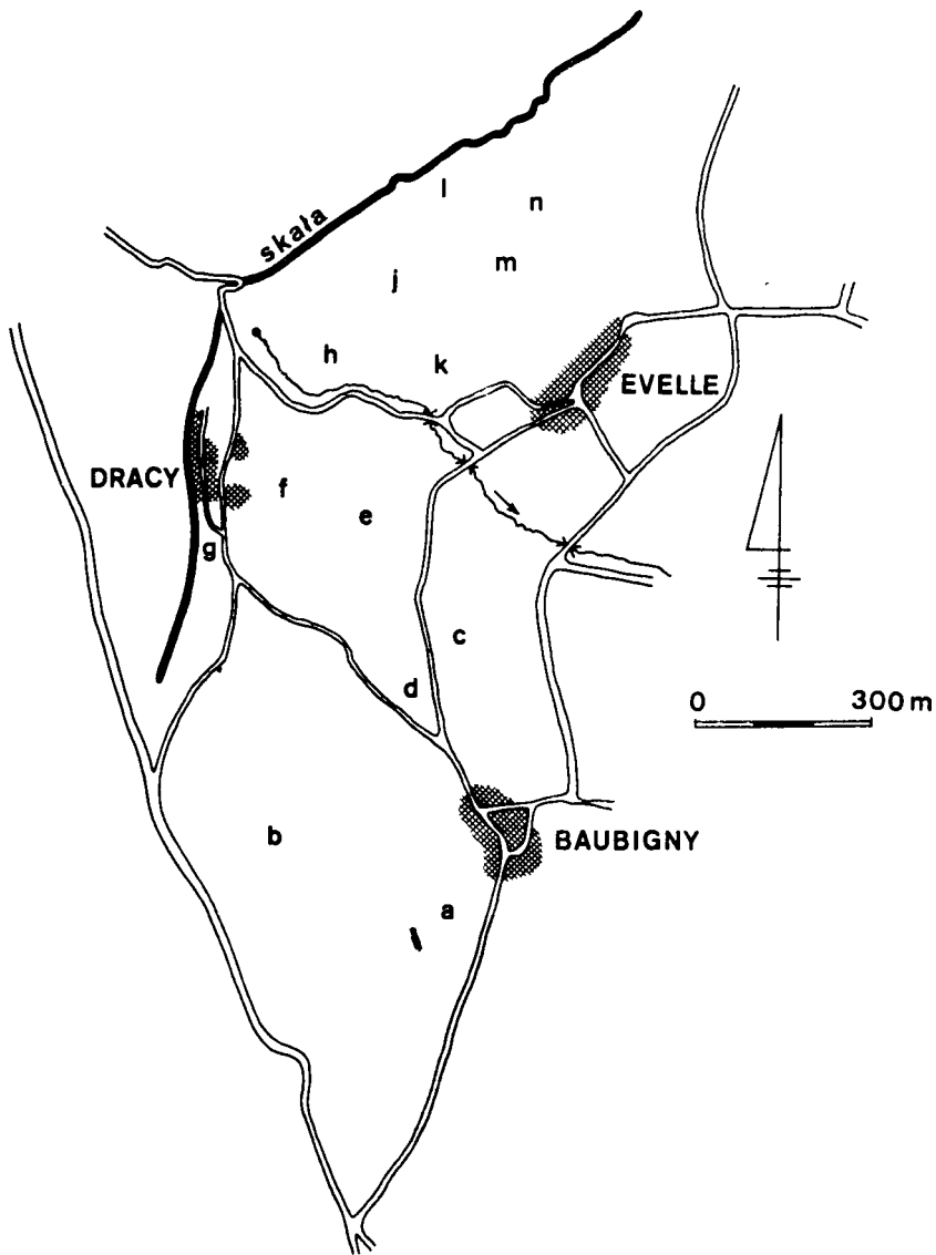
Ryc. 5. Podstawowe parcele wokół Dracy według kadastru w przeryszie z 1953 r. a — „Derrière Baubigny”, b — „Aux Craies”, c — „La Corvée”, d — „Derrière le Chapitre”, e — „En Bras”, f — „Les Champs de Bras”, g — „Sous les Roches de Baubigny”, h — „En Dréché”, j — „Sous le Bois Michel”, k — „Sur Evelle”, l — „Les Trois Roches”, m — „En Moulinot”, n — „Sur le Chemin Neuf”. Rysowała Emilia Grabarczyk
