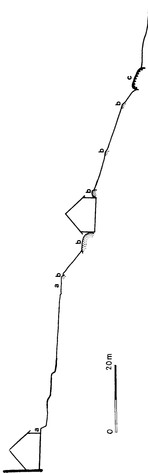
Ryc. 4. Przekrój przez północną część Dracy oraz przez terasy pól przyzagrodowych
