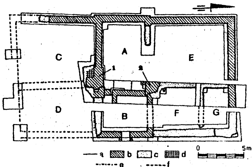
Rys. 9. Burzenin, gm. loco, woj. Sieradz, stanowisko 3. Rzut odsłoniętych reliktywów dworu murowanego (XVI-XVIII w.). A - najstarsza partia dworu, 1 - tzw. mur 1; 2 - tzw. mur 2; B - piwnica wschodnia (tzw. obiekt 1) - I faza rozbudowy; C, D - piwnice południowe; E, F, G - pomieszczenia północnej partii dworu - II faza rozbudowy; a - granice wykopów, b - mur ceglany, c - partia fundamentowa z kamienia, d - posadzka z płytek ceglanych, e - negatyw fundamentów, f - domniemany przebieg murów
