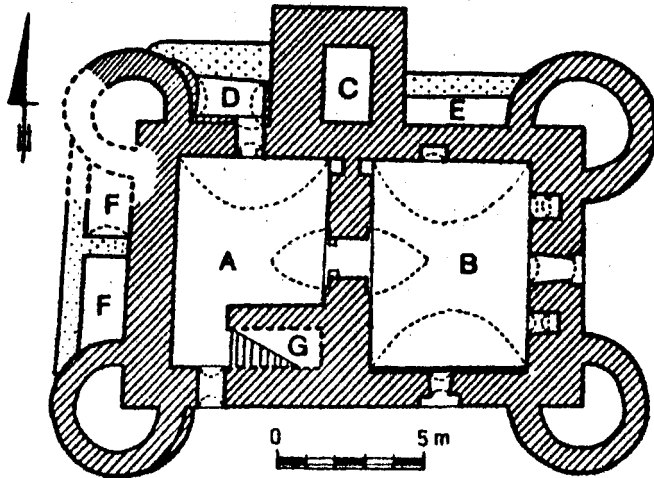
Rys. 11. Żuków, gm. Wieniawa, woj. Radom, stanowisko 1. Rzut reliktyw dworu murowanego z XVI-XVIII w. na poziomie przyziemia. A - piwnica zachodnia, B - piwnica wschodnia, C - ryzalit północny, D - tzw. aneks północno-zachodni, E - tzw. aneks północno-wschodni, F - tzw. aneks zachodni, G - pion komunikacyjny (schody kamienne)
