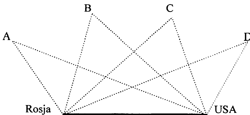
Ryc. 3. Miękkie kondominium empatyczne Fig. 3. Soft empathic condominium
