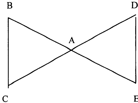
Ryc. 5. Triada triad połączonych – A jest zwnikiem triad Fig. 5. The triad of combined triads: A is the connector of triads
