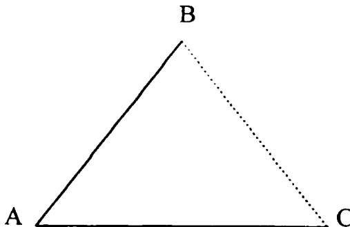
Ryc. 2. Triada niestabilna: C jako wróg przyjaciela B jest przyjacielem dla A Fig. 2. Unstable triad: C as an enemy of B's friend is A's friend
