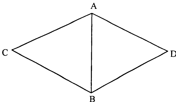
Ryc. 6. Inny typ triady połączonej – A i B zwornikami triad Fig. 6. Another type of the combined triad: A and B are triad connectors
