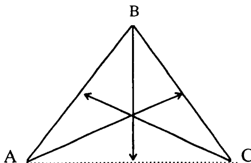
Ryc. 4. Triada niestabilna: C jako przyjaciel przyjaciela B jest wrogiem dla A Fig. 4. Unstable triad: C as a friend of B's friend is A's enemy
