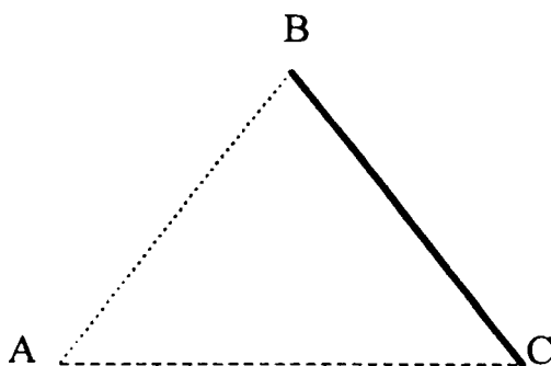
Ryc. 7. Triada, w której stosunki nie są oceniane w sposób binarny: stosunki B z C są najlepsze, A z B gorsze, a A z C najgorsze
