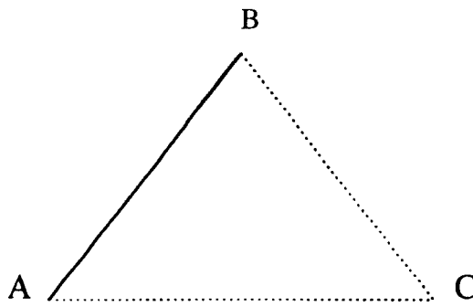
Ryc. 1. Triada stabilna: C jako wróg przyjaciela B jest wrogiem dla A Fig. 1. Stable triad: C as an enemy of B's friend is A's enemy
