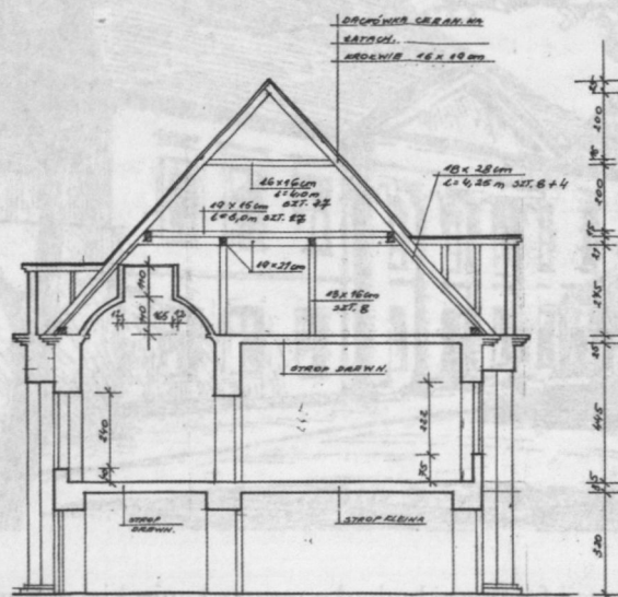
PRZEKRÓJ A-A
