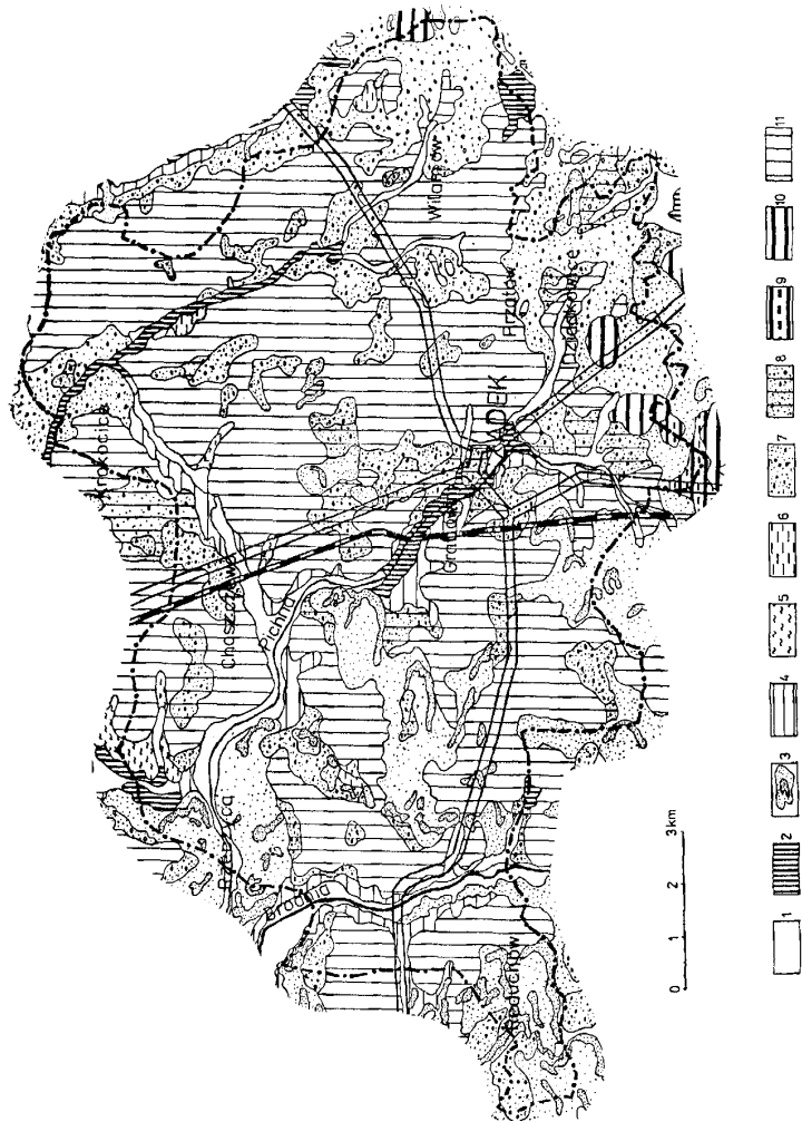
Rys. 2 Słukie geologiczne, powierzchniowy okolic Szadku (na podstawie: Baliński 1990, 1992, Bezkowska 1995, 1993, Klatkova 1985, 1988, Klatkova i in. w druku; zmieniłone)
