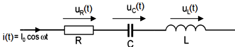
Obrázok 1. Sériové zapojenie obvodu RLC
