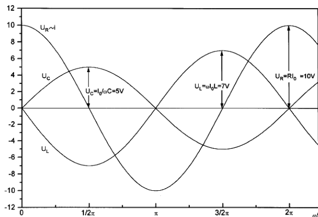
Obrázok 2. Časové priebehy napätí u_R(t) , u_C(t) a u_L(t)
