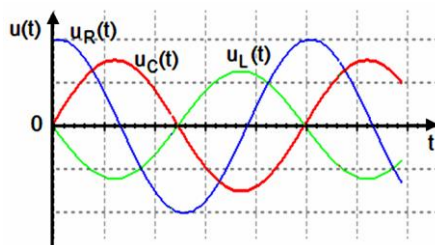
Obrázok 3. Namerané priebehy harmonických napätí u_R(t) , u_C(t) a u_L(t) na prvkoch RLC
