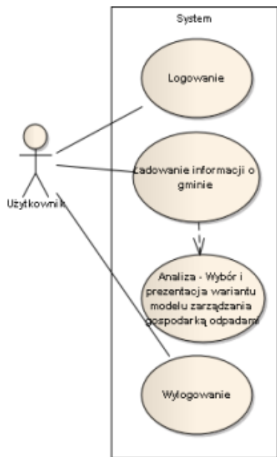
Rys. 1. E-aplikacja do wyboru modelu zarządzania gospodarką odpadami
