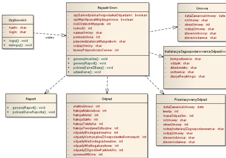
Rys. 2. Diagram klas
