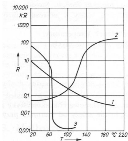
Rys. 5. Charakterystyka rezystancyjno-temperaturowa termistorów (1-NTC, 2-PTC, 3-CTR) [Gajek, Juda 2009]
