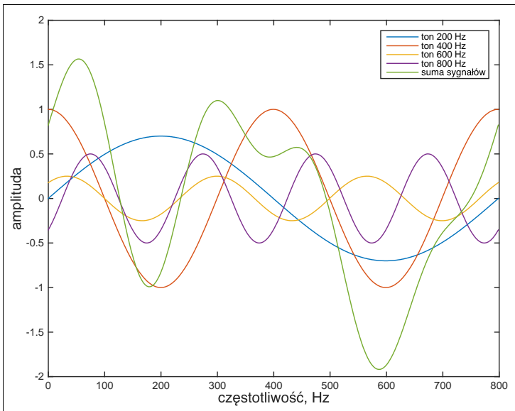
Wykres 1. Tony o częstotliwościach 200, 400, 600 i 800 Hz i ich suma
