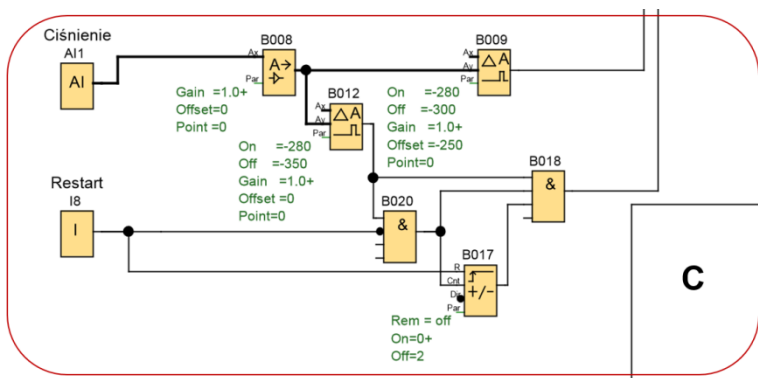
Rysunek 5. Moduł kontroli wartości i sterowania ciśnieniem
