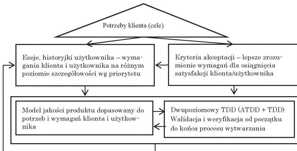
Rys. 3. Sterowanie jakością za pomocą iteracyjnego modelu jakości, dopasowanego do potrzeb klienta i użytkownika za pomocą testowania akceptacyjnego i deweloperskiego, wyprzedzającego pisanie kodu produkcyjnego
