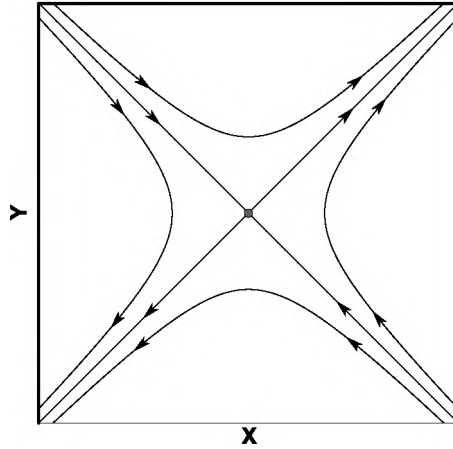
Rys. 3. Portret fazowy siódła dwuwymiarowego
