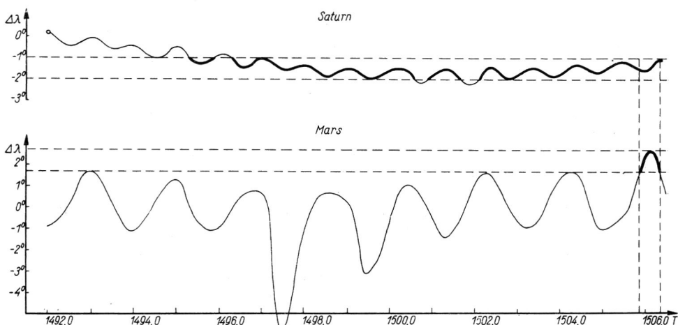
Ryc. 2. Poprawki długości planet w Tablicach alfonsyńskich
