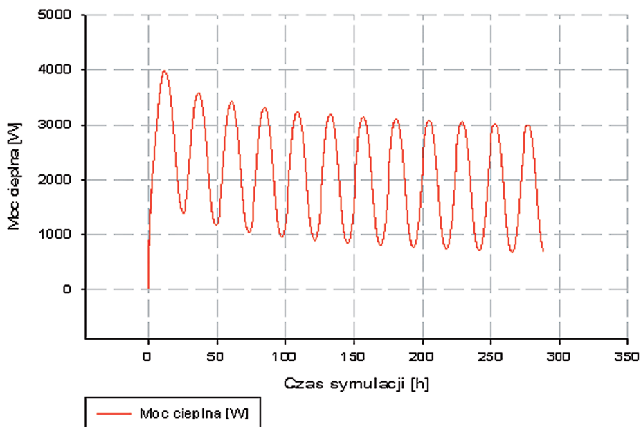
Ryc. 9. Moc ciepła oddawana przez ściankę zewnętrzną rury zewnętrznej do gruntu
