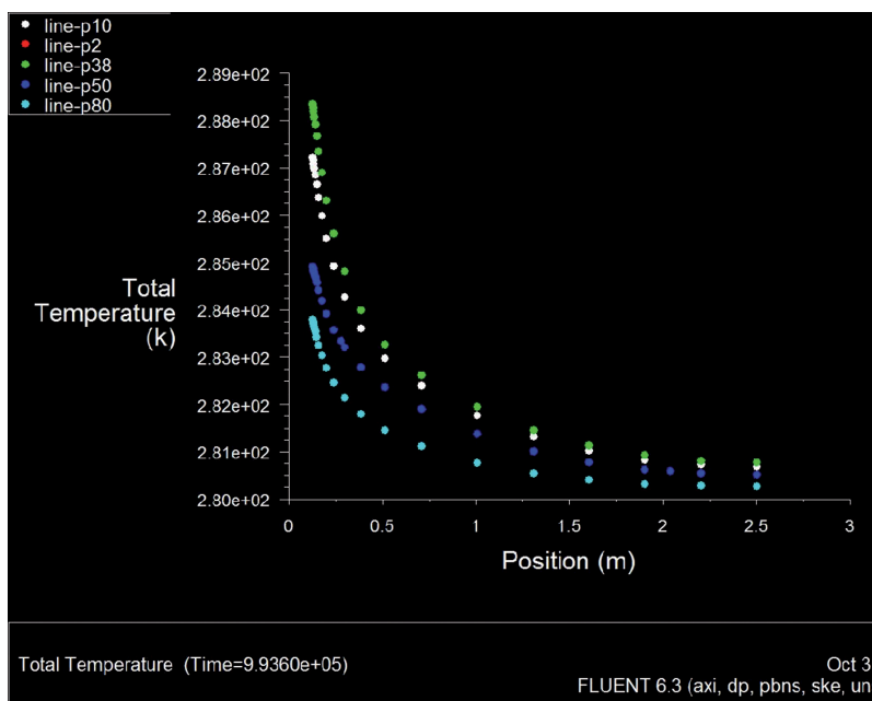
Ryc. 11. Rozkład temperatury w funkcji promienia
