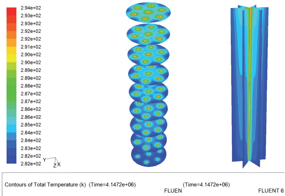
Ryc. 22. Przekroje temperatury gruntu co 10 m i obraz pola 3D – po upływie 48 dni
