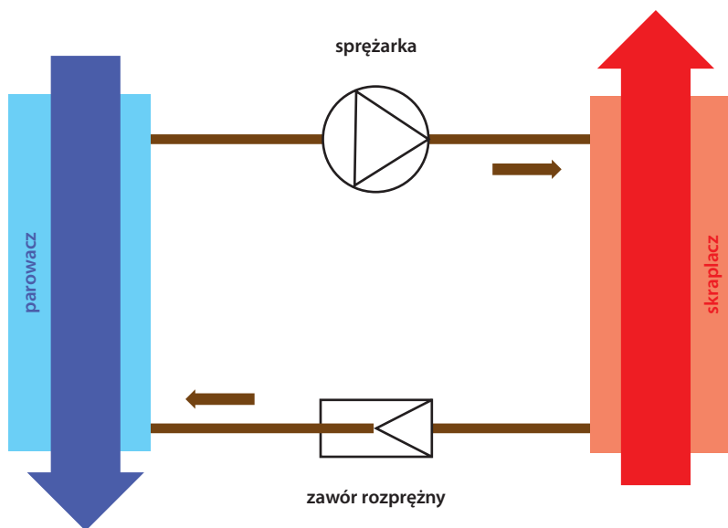
Rys. 3. Uproszczony schemat działania pompy ciepła
