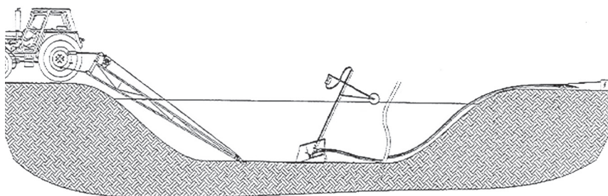
Ryc. 4. Schemat przeciągania liną odmularki po dnie zbiornika wodnego za pośrednictwem wciągarki zainstalowanej na wysięgniku mocowanym do ciągnika
