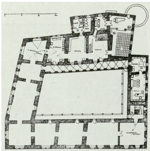
6. Zamek Blansko, plan parteru po rekonstrukcji (fot. L. Lacina)
