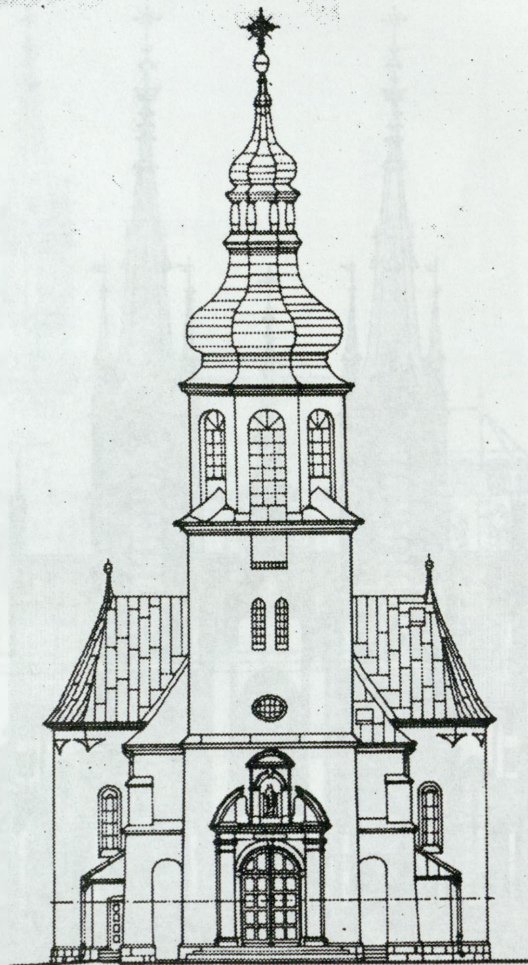
13. Blonie Łęczyżskie 1906, pomiar fotogrametryczny 1986 13. Blonie Łęczyżskie 1906, photogrammetric measurement 1986
