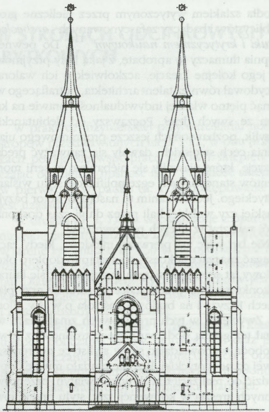
15. Kulesze Kościelne 1911 wg proj. realizacyjnego 15. Kulesze Kościelne 1911 according to a realisation project
