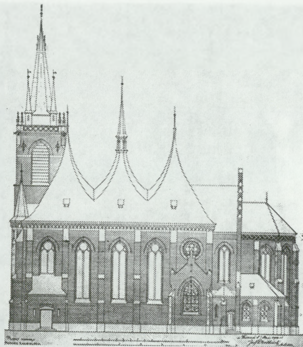
6. Popowo Kościelne, elewacja boczna wg proj. wstępnego 6. Popowo Kościelne, side elevation according to an initial project
