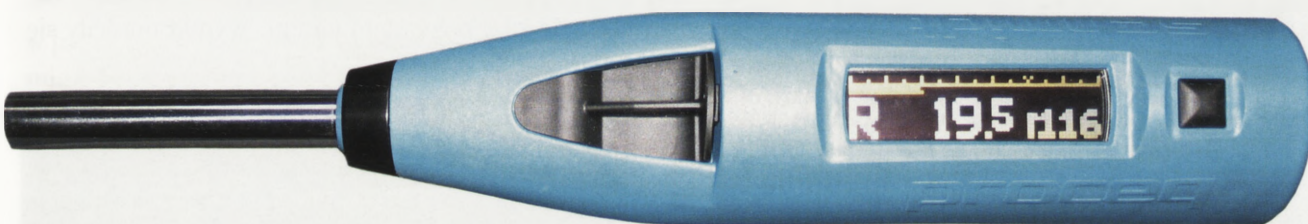
3. Młotek Silver Schmidt firmy Proceq. Fot. P. Filipowicz. 3. A Silver Schmidt hammer made by Proceq. Photo: P. Filipowicz.
