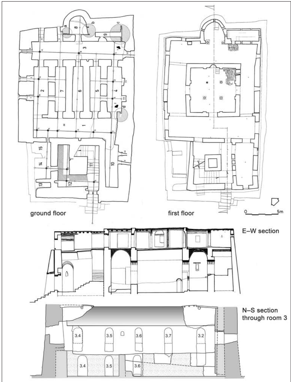
Fig. 4. The Mosque Building (archival documentation, 1980) (P.M. Gartkiewicz, B. Kubicz; S. Medeksza; W. Godlewski, S. Maślak; PCMA Archives)
