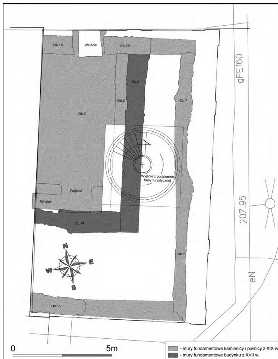
Ryc. 3. Chełm, ul. Przechodnia. Plan murów odkrytych w czasie badań. Kamienica z piwnicą (ob. 1A, 1B, 2, 3, 7, 15) z XIX w. i fragment budynku z XVII w. (ob. 4, 14). Oprac. S. Gołub. Rys. i oprac. komp. R. Ratajczak
