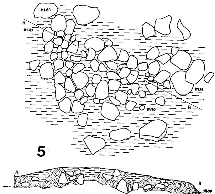
Ryc. 12. Ostrów Lednicki, st. 1 – 2. Typy palenisk. 1 — wklęsłe (zagięzione) bez obstawy kamiennej, 2 — wklęsłe (zagięzione) z podkładem kamiennym i płytą glinianą, 3 — zagięzione z obstawą kamienną, 4 — wypukłe bez podkładu kamiennego, 5 — wypukłe z podkładem kamiennym
