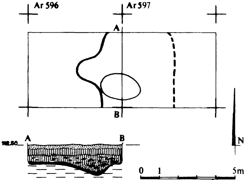
Ryc. 11. Rzut poziomy i przekrój półziemianki z korytarzem z podgrodzia
