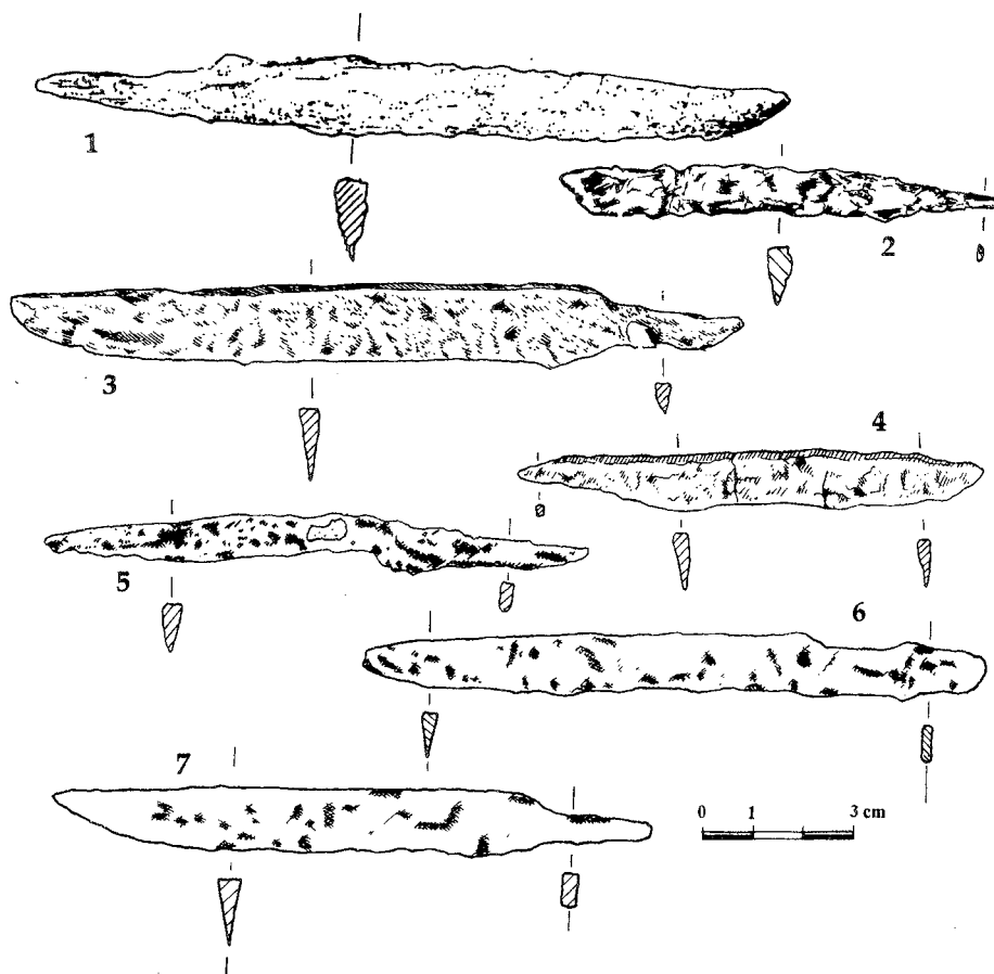
Ryc. 18. Noże z grobów osobników o nieokreślonej płci — typ Ia: 1 — 5/84; 3 — 52/94; typ Id: 2 — 20/97; 4 — 63/94; typ Ie: 5 — 1/92; typ If: 6 — 6/95; 7 — 80/95.
