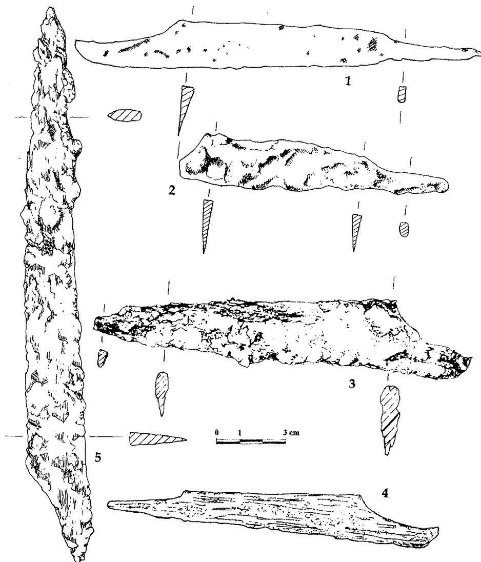
Ryc. 10. Noże typ VIa z grobów mężczyzn: 1 — 93/95; 2 — 75/94; 3 — 4/86; 4 — 2/64; 5 — 31/97.
