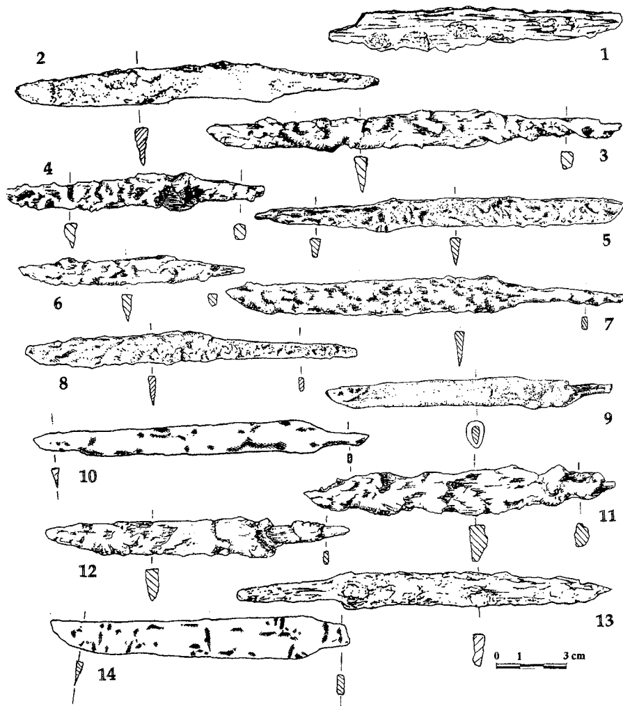
Ryc. 4. Noże typ Ia z grobów mężczyzn: 1 — 1/64; 2 — 6/84; 3 — 40/97; 4 — 58/97; 5 — 82/94; 6 — 37/96; 7 — 9/94; 8 — 62/94; 9 — 75/97; 10 — 56/95; 11 — 60/95; 12 — 30/97; 13 — 13/77; 14 — 36/95.
