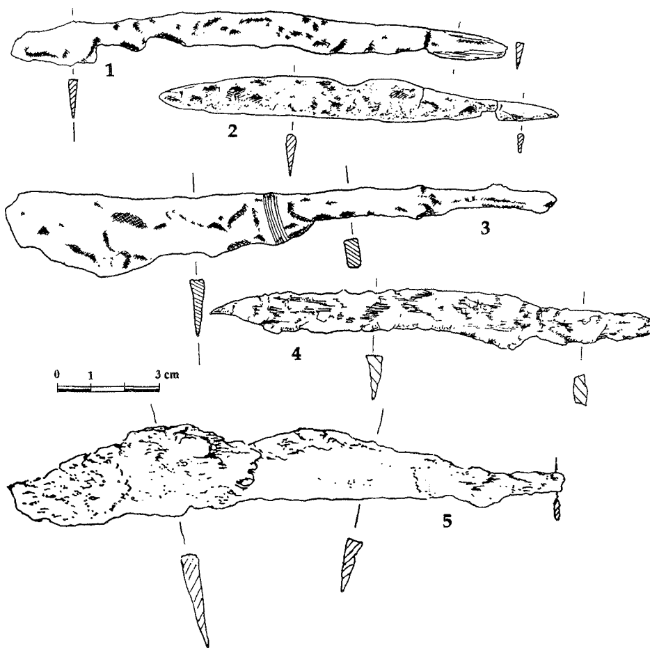
Ryc. 12. Noże z grobów mężczyzn — typ IV?: 1 — 4/95; 2 — 41/94; typ V: 3 — 2/95; typ VII: 4 — 59/97; typ IIId – IV?: 5 — 1/91.
