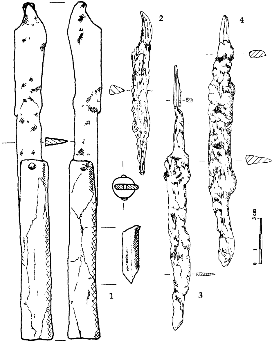
Ryc. 11. Noże z grobów mężczyzn — typ VIa: 1 — 82/95 i typ VIb: 2 — 7/77; 3 — 23/97; 4 — 28/97.
