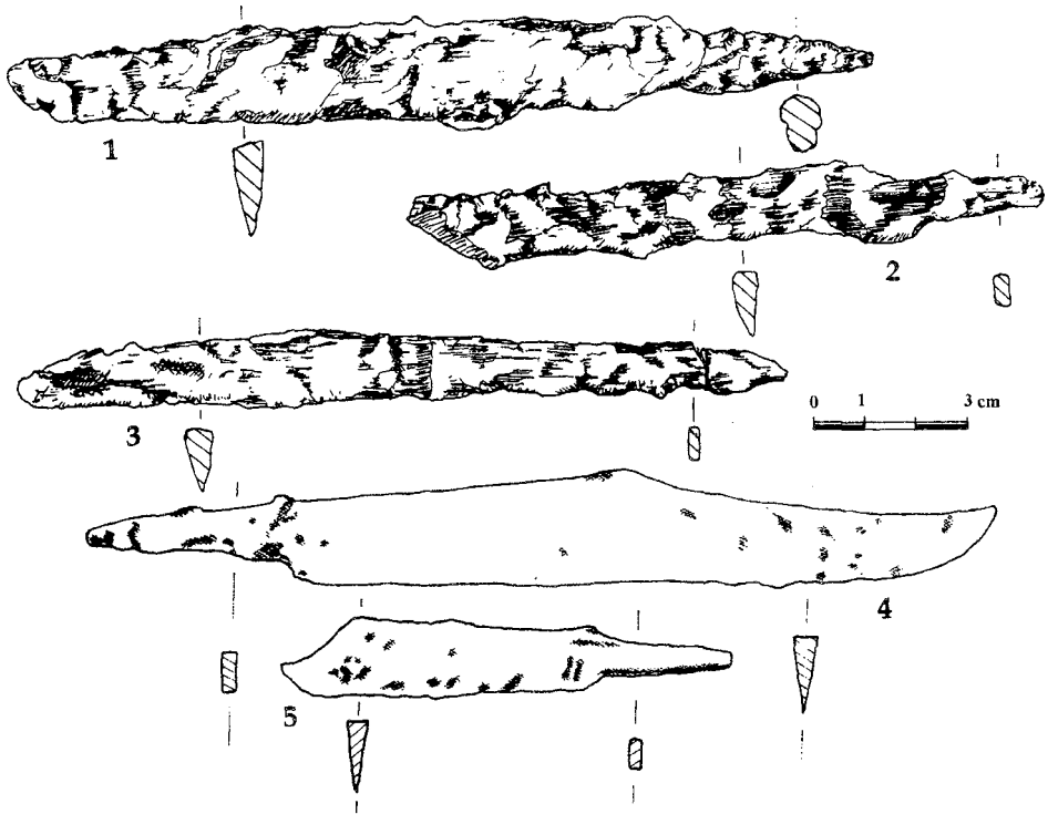
Ryc. 19. Noże z grobów osobników o nieokreślonej płci — typ IIb: 1 — 45a/97; typ IIc: 2 — 75/97; typ IV: 3 — 76/97; typ VIa: 4 — 71/95; 5 — 78/95.
