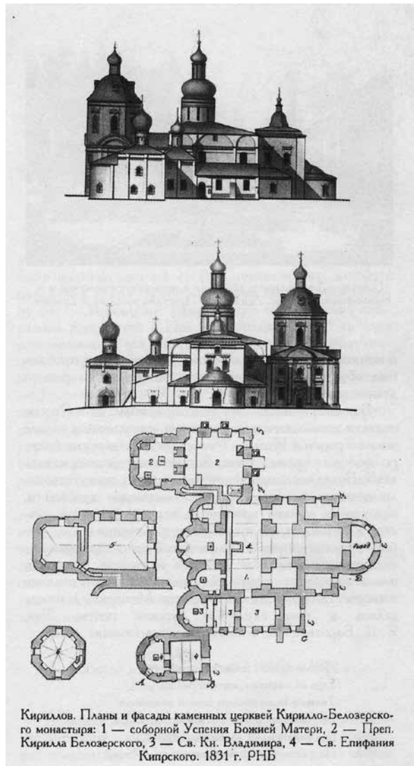
Il. 3. Plany i fasady cerkwi monastynu Kirillo-Belozerskiego wykonane w związku z ukazem cara Mikołaja I w 1831, wg Щенков (2002: 47)
